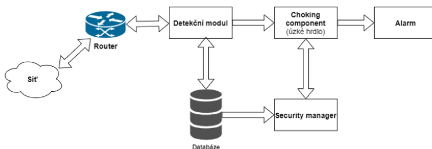
obrázek č. 6 – Architektura Source-end defense mechanism, zdroj: [28]
