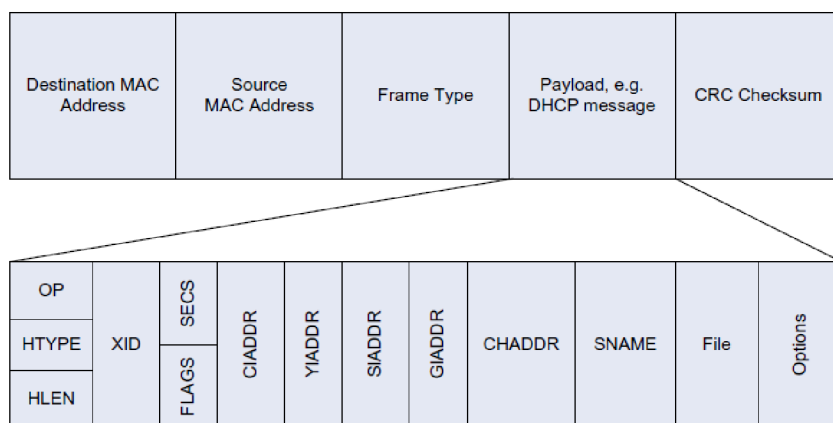
obrázek č. 16 – Ethernetový rámec s paketem DHCP, zdroj: [11]
