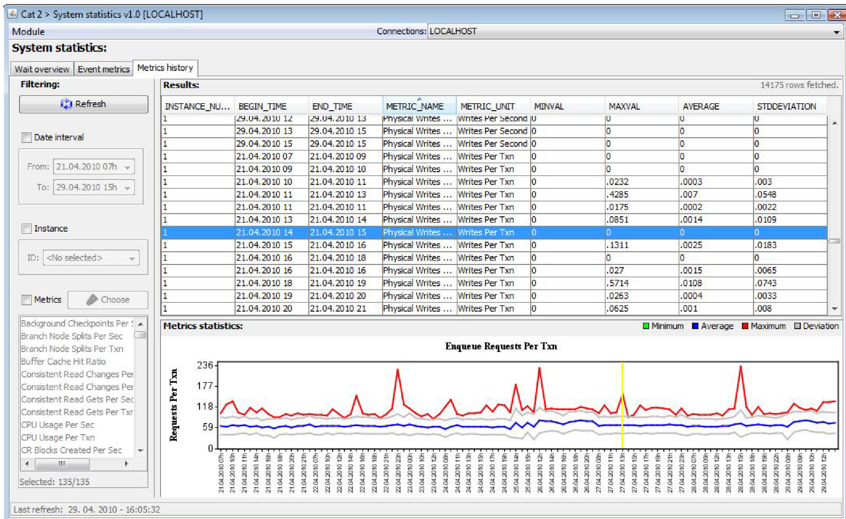
Obrazek C.9: Běžící modul „System Statistics“ – jeho část zobrazující historii metrik.
