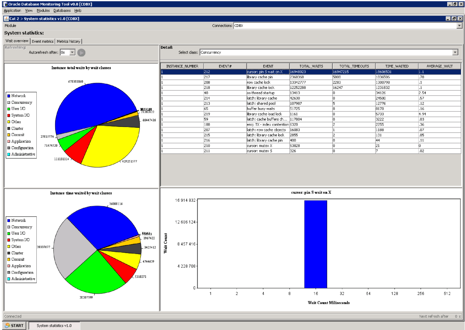
Obrázek 6.1: Úzké místo produkční databáze, které bylo zjištěno vytvořenou aplikací.
