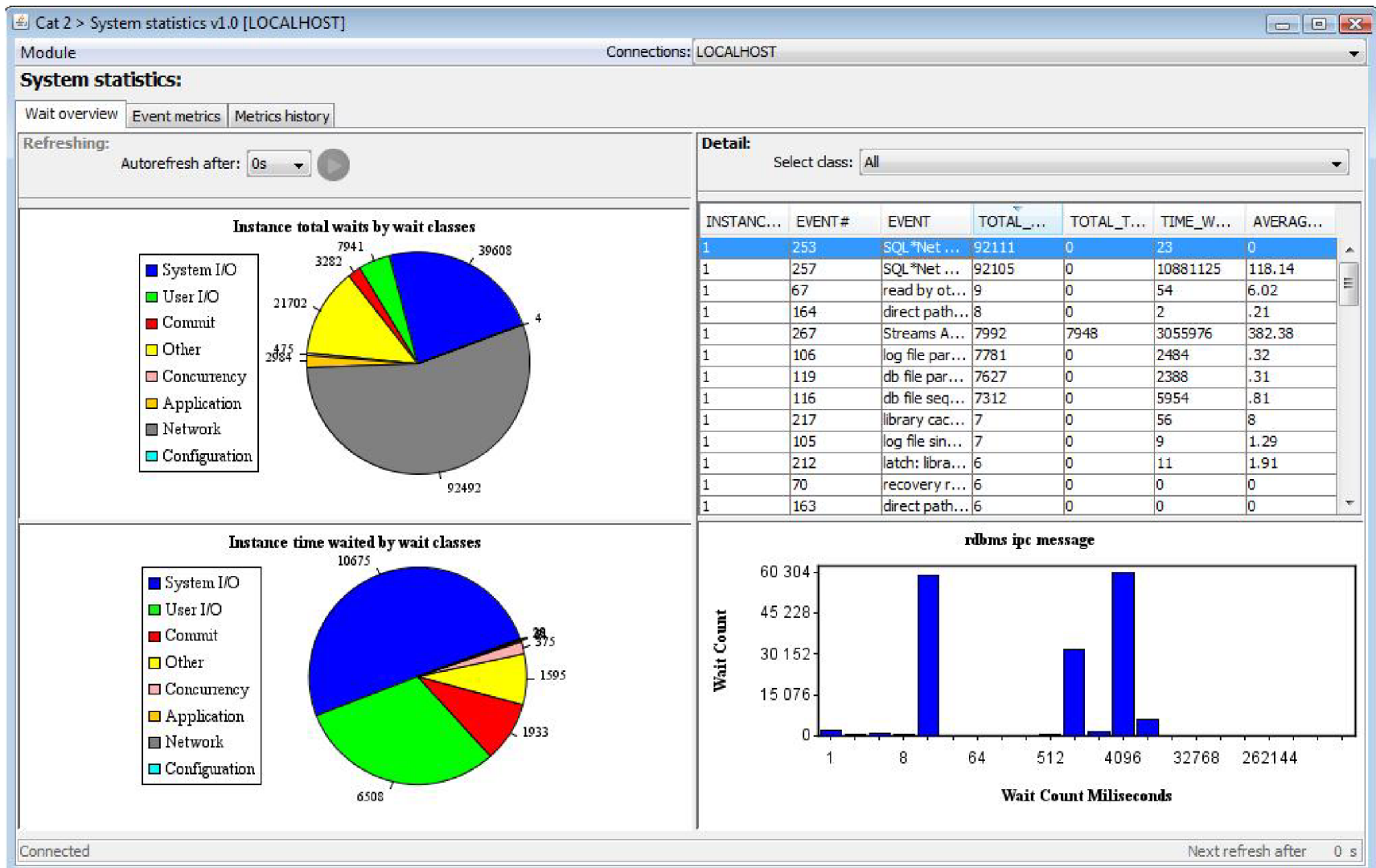
Obrázek C.6: Běžící modul „System Statistics“ – jeho část zobrazující přehled Wait Inter-
