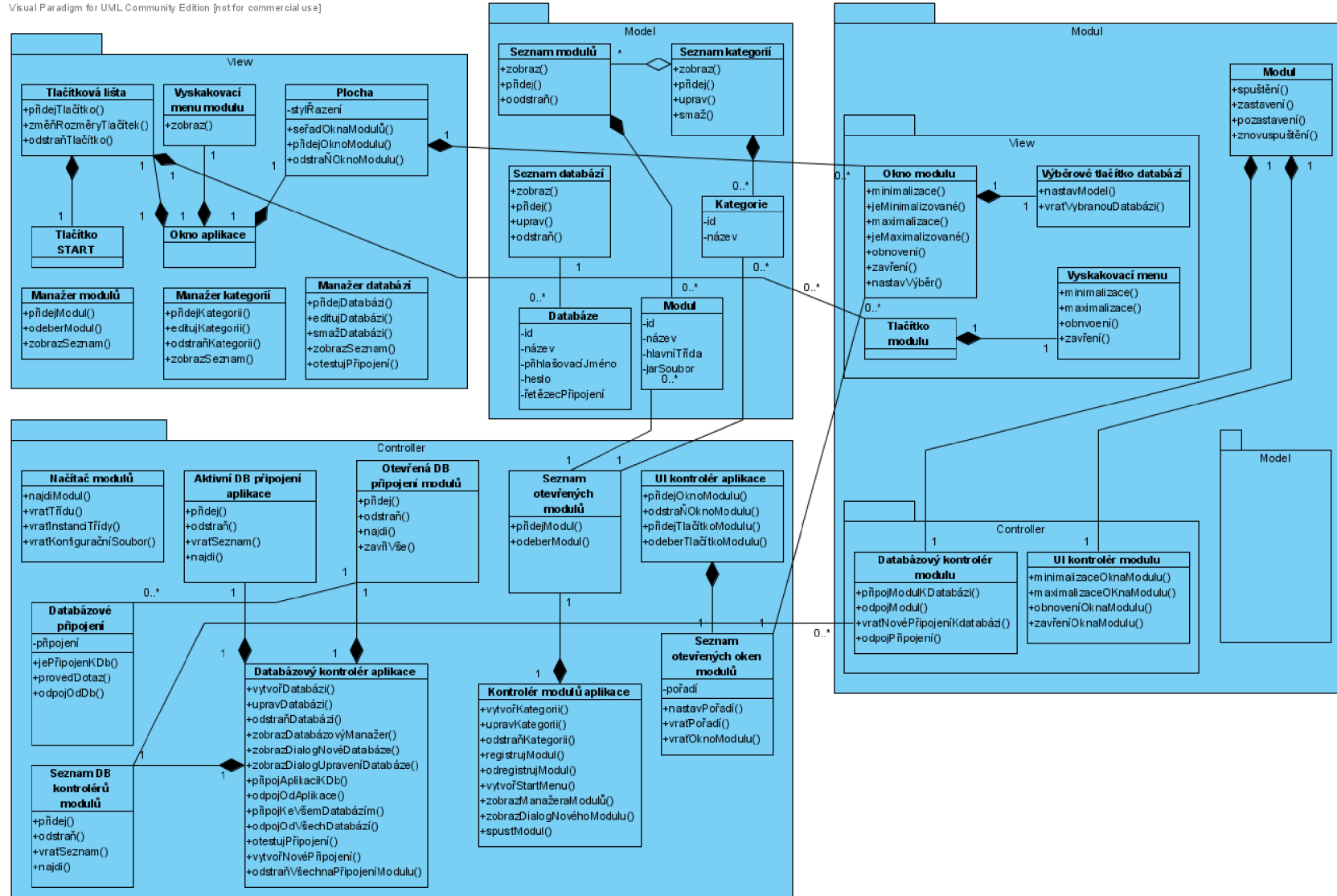
Obrázek 3.3: Diagram tříd
