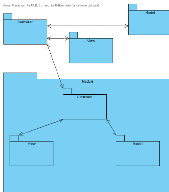
Obrázek 3.2: Diagram balíků
