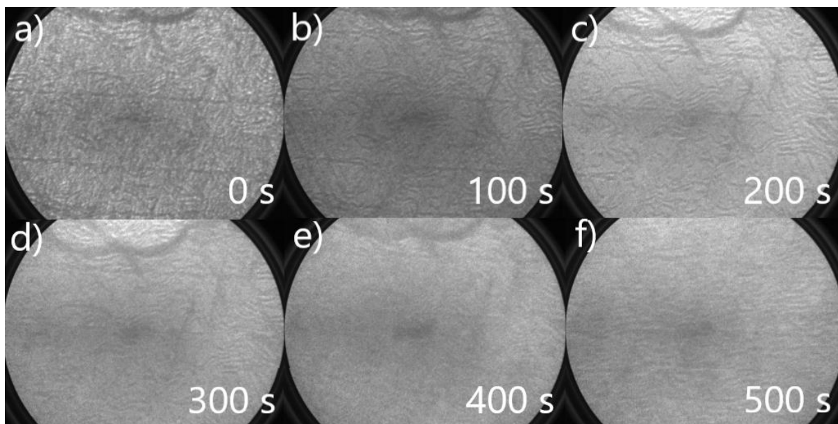
Obrázek 5.5: Časový průběh změny struktury substrátu ( 3 \mu\text{m} ). Obrázky a), b) a c) byly pořízeny při ohřevu na 215 \text{ }^\circ\text{C} , je na nich patrný mírný úbytek teras a tmavých míst odpovídajících fosforu. Obrázky d) a e) byly pořízeny po stabilizaci teploty a předchozí děje zde probíhají zrychleně. Obrázek f) zobrazuje již zcela porušenou strukturu povrchu.
