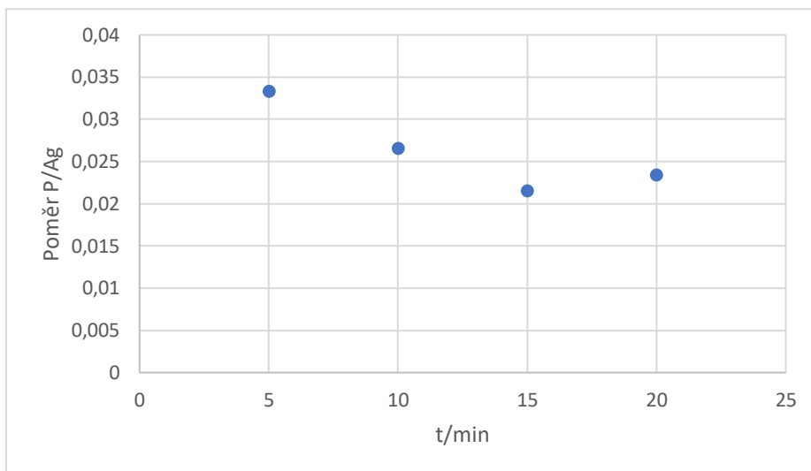
Obrázek 5.3: Poměr ploch píků Ag 3d 3/2 a P 2p 3/2 v závislosti na době depozice. Pětiminutová a desetiminutová depozice obsahuje největší množství fosforu, zřejmě z důvodu žíhání za nižší teploty (100 °C) než u následujících (150 °C).
