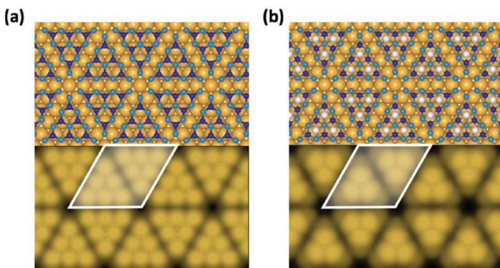
Obrázek 2.3: Teoretický model modrého fosforenu s odpovídajícím STM snímkem. a) Horní část zobrazuje modelové trojúhelníkové útvary složené ze 16 atomů fosforu. Zvrásnění fosforenu vede k vyzdvihnutí některých atomů (podle obrázku 2.1), které můžeme pozorovat pomocí STM, jak můžeme pozorovat na dolním obrázku. b) Trojúhelníkový útvar složeny ze 16 atomů fosforu je doplněn o fosforový trimer. Ten „zastíní“ spodní vrstvy a na STM snímku pozorujeme v rámci trojúhelníku už pouze tyto tři atomy. Převzato z [9].
