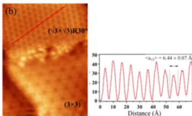
Obrázek 1.5: Měření elektronové hustoty stavů pomocí STM. Vzdálenost dvou minim je (6,44 \pm 0,07) Å a odpovídá mřížkové konstantě silicenu – a_{ML} = (6,477 \pm 0,015) Å. Převzato z [7].
