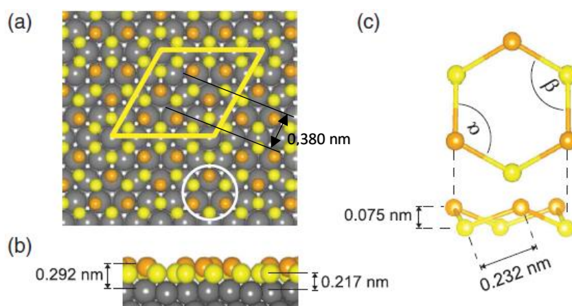
Obrázek 1.1: Struktura silicenu. a) elementární buňka – oranžovou barvou označené atomy křemíku jsou usazeny na atomech stříbra označených šedou, „žluté“ atomy křemíku se usazují mezi nimi, je zde patrná šestiúhelníková struktura silicenu, v níž jsou atomy od sebe vzdáleny 0,380 nm b) pohled v řezu – zvlněná křemíková vrstva dává vzniknout dvěma atomovým rovinám s rozdílnými vzdálenostmi od povrchu substrátu c) šestiúhelníkový prstenec silicenu – délka vazby mezi křemíkovými atomy je 0,232 nm, vzájemná vzdálenost obou atomových rovin je 0,075 nm. Převzato z [5].
