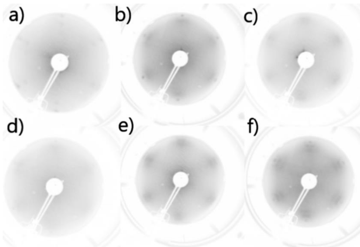
Obrázek 5.2: Difrakční obrazce po depozici s teplotou substrátu 260 °C a následném vyžhání. V a) depozice trvala 15 minut a vzorek byl žhán 10 minut na 155 °C, difrakční body zde připomínají ty u Ag (111), v b) se jednalo o pětiminutovou depozici a desetiminutové žhání vzorku na 100 °C, v c) a d) se zvýšila doba depozice na 10 a 20 minut, v e) difrakční obrazec vzorku z d) po dalším desetiminutovém žhání, tentokrát na 150 °C, objevil se zde náznak složitějšího difrakčního obrazce než u Ag (111), v f) se jednalo opět o patnáctiminutovou depozici s desetiminutovým žháním na 150 °C, v tomto případě bylo možno rozeznat vícero difrakčních bodů než by odpovídalo substrátu.
