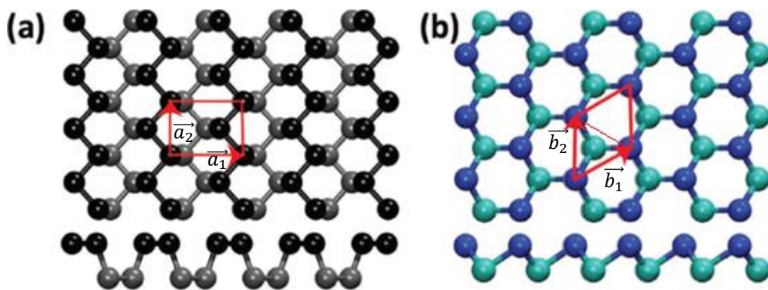
Obrázek 2.1: a) Struktura černého fosforu (tmavé atomy označují vyšší atomovou rovinu, světlé atomy označují nižší atomovou rovinu). Horní obrázek popisuje elementární buňku s primitivními vektory |\vec{a}_1| = 0,437 \text{ nm} a |\vec{a}_2| = 0,331 \text{ nm} . Spodní obrázek ukazuje pohled v řezu. b) Struktura fosforenu (modré atomy označují vyšší atomovou rovinu, zelené atomy označují nižší atomovou rovinu). Horní obrázek popisuje elementární buňku s primitivními vektory |\vec{b}_1| = |\vec{b}_2| = 0,328 \text{ nm} . Spodní obrázek ukazuje pohled v řezu. Převzato z [9].
