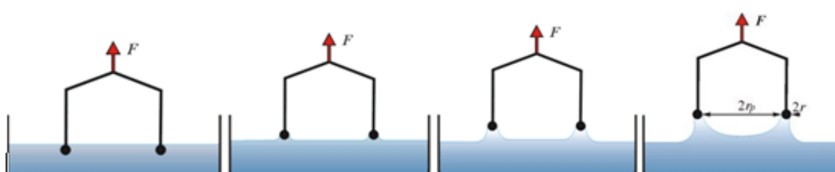
Obrázok 3: Znázornenie priebehu procesu odtrhávania prstenca [9].
