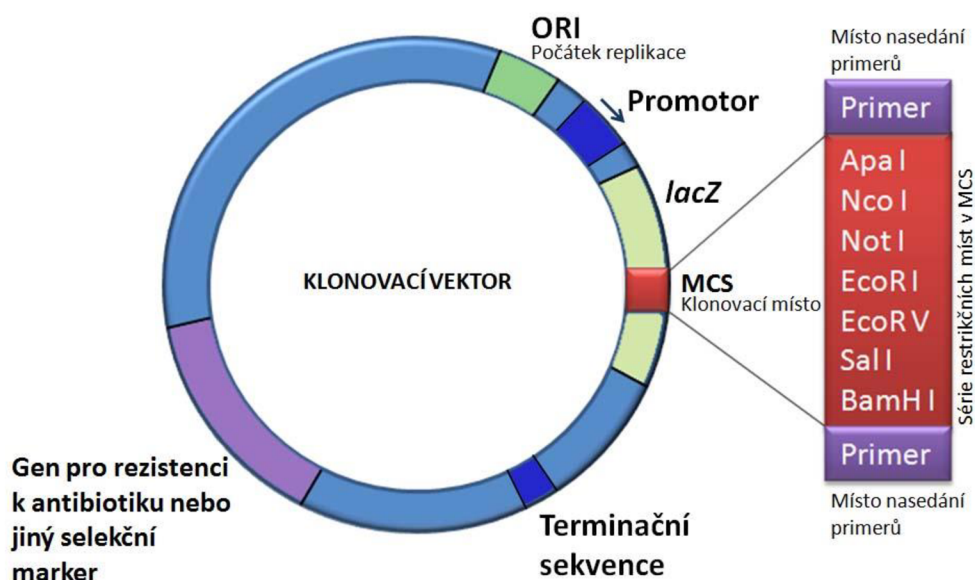
Obrázek 2: Klonovací vektor [5]
