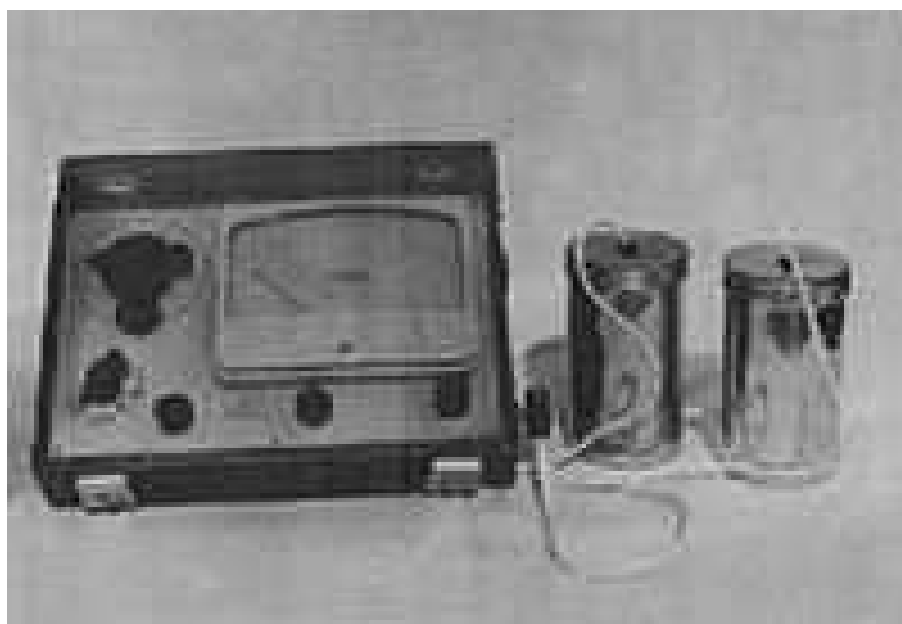
Původní provedení e-metru v dřevěné krabičce
