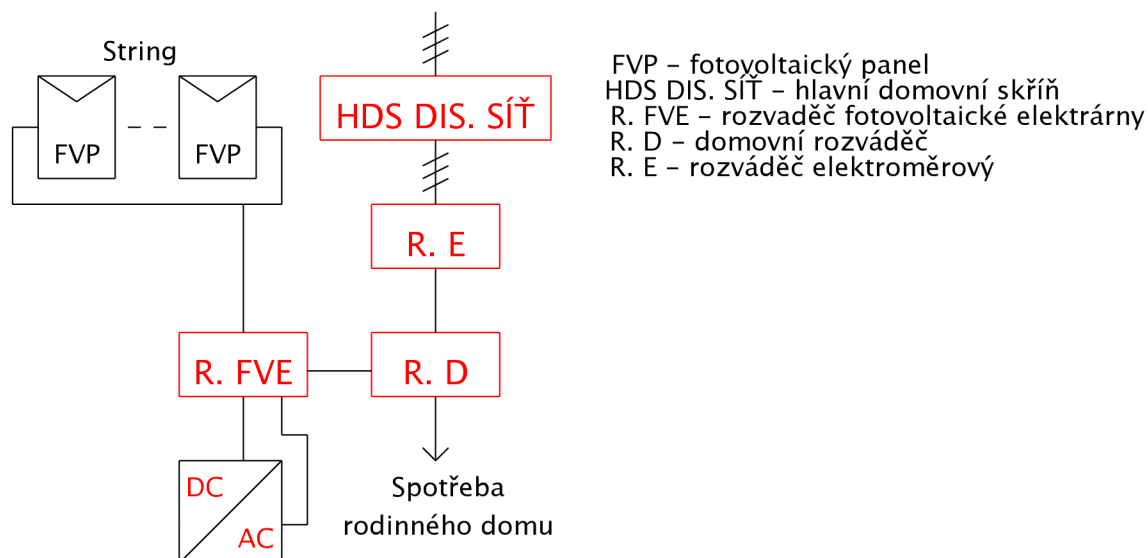
Obrázek 4-1 Blokové schéma zapojení poloostrovního energetického systému pro zelený bonus bez akumulace elektrické energie [23]
