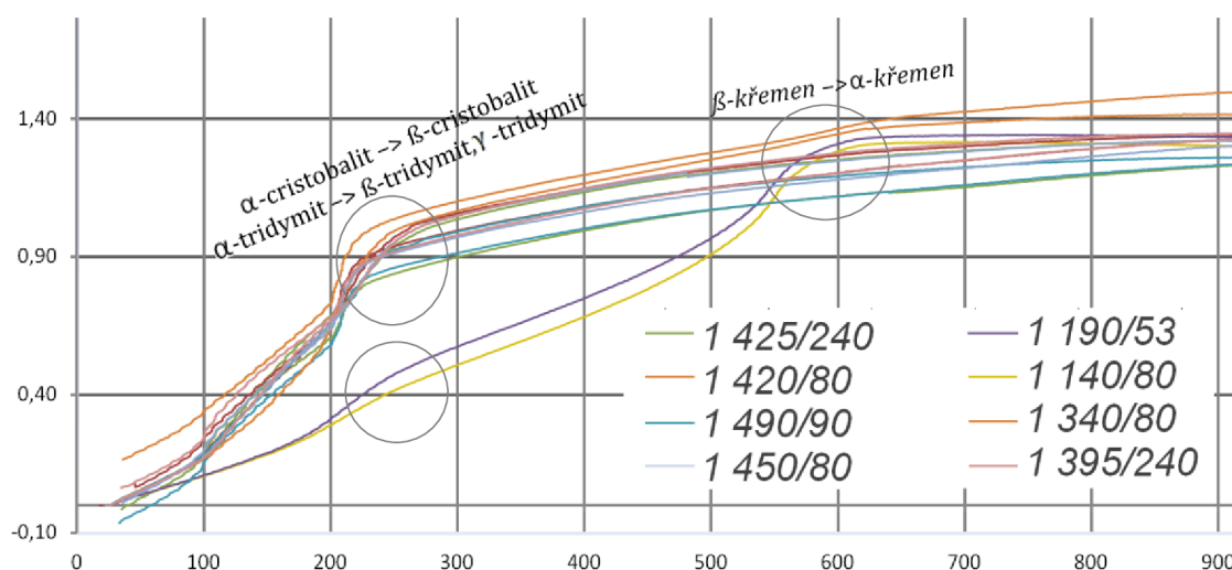
Obrázek 34: Detail délkových změn do 900 °C
