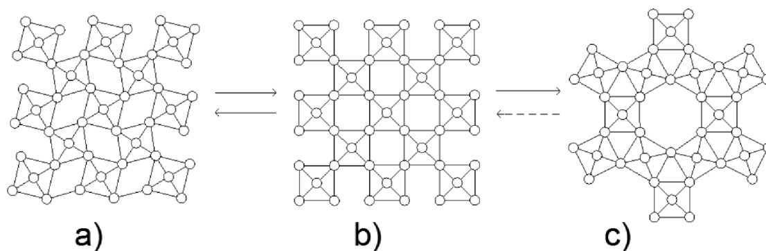
Obrázek 11: Strukturní schéma přeměn modifikací \text{SiO}_2 [22]
