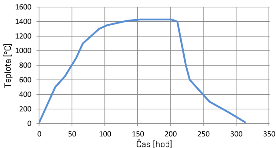
Obrázek 1: Charakteristická palicí křivka [12]
