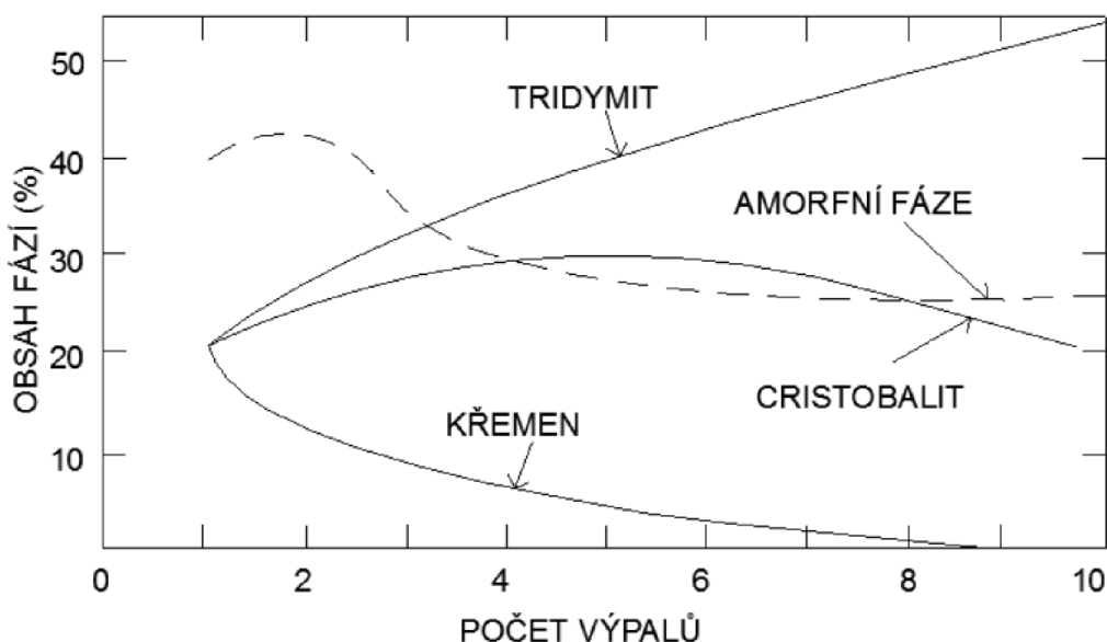
Obrázek 3: Změna fázového složení dinasů při opakovaných výpalech [13]
