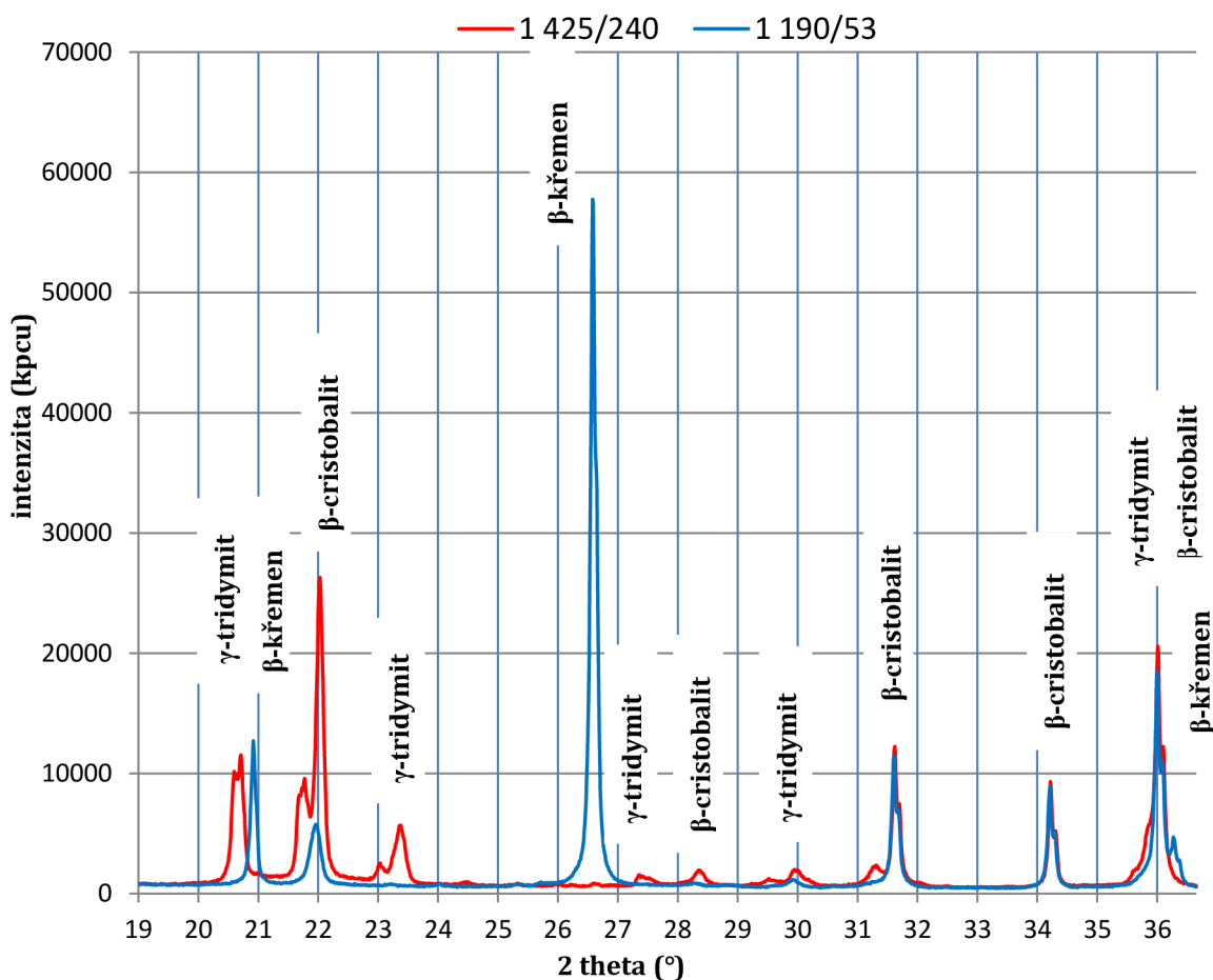
Obrázek 30: Difraktogram zkušebních vzorků 1 425/240 a 1 190/53
