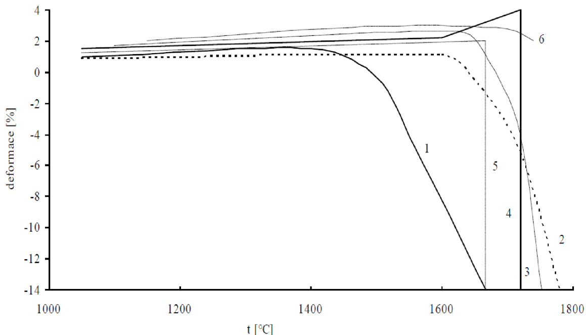
Obrázek 21: Deformační průběhy žárovzdorných materiálů. 1-šamot, 2-silimanit, 3-chrommagnezit, 4-sklářský dinas, 5-koksárenský dinas, 6-magnezitochrom [19]
