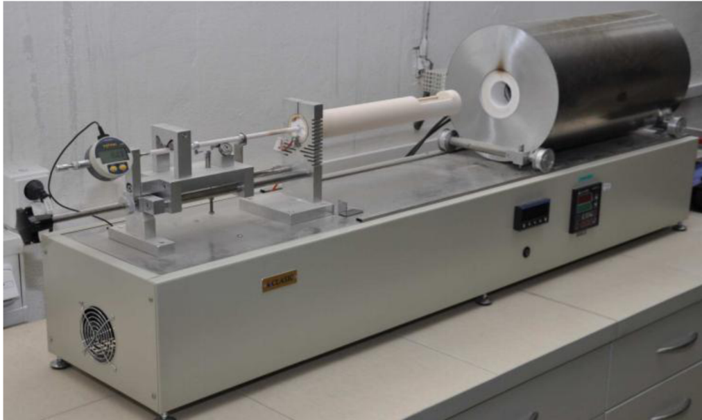
Obrázek 19: Příklad pro stanovení DKTA [30]
