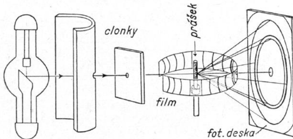
Obrázek 17: Uspořádání práškové rentgenové difrakční analýzy [5]
