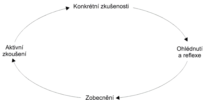
Obr. 1 Kolbův cyklus
