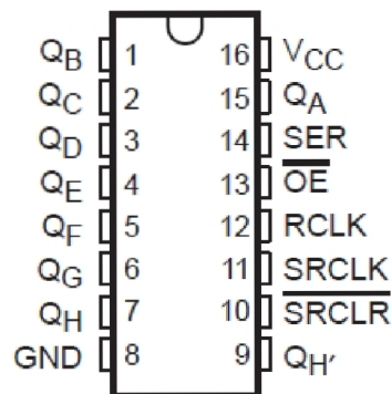
obrázek 7: posuvný registr
