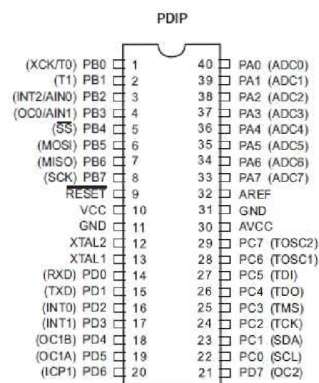
obrázek 6: ATMega 16 [5]
