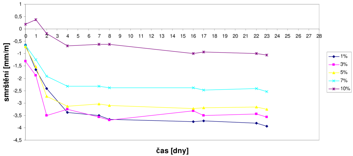
Obrázek 26 Závislost smrštění vzorků na čase – Hlína J
