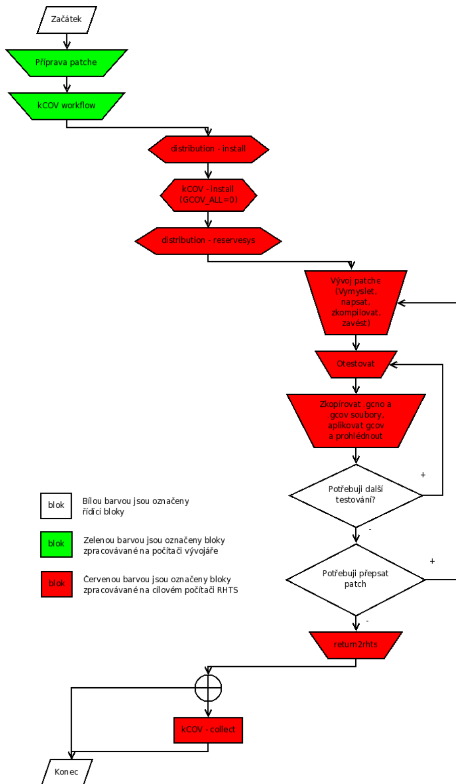
Obrázek 4.5: Proces vývojáře
