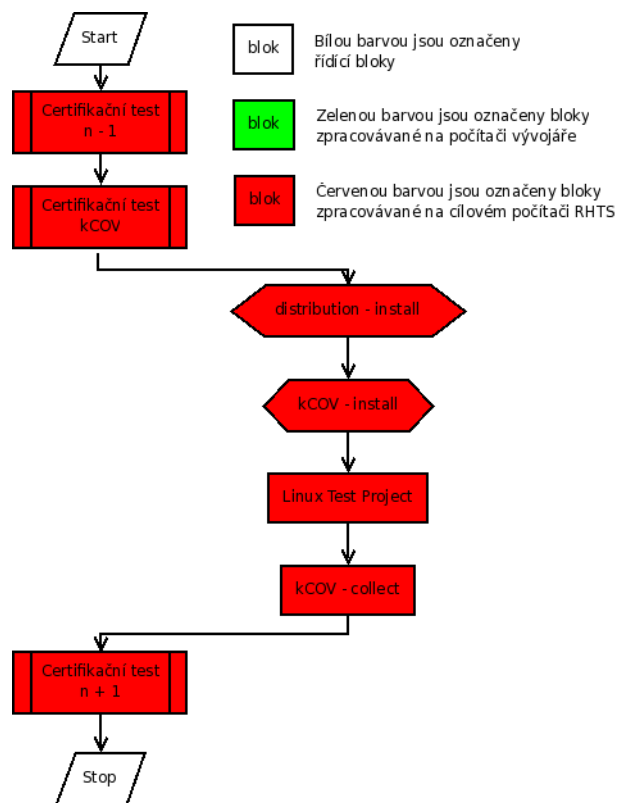
Obrázek 4.3: Proces certifikace
