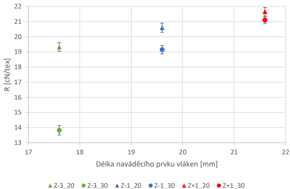
Graf 9 Vliv délky naváděcího prvku na poměrnou pevnost přízí
