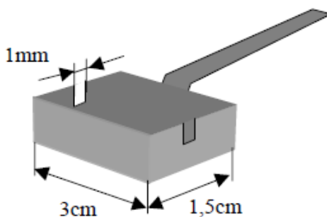
Obrázek 14 Vanička pro zalévání příze do směsi včelího vosku a parafínu [45]
