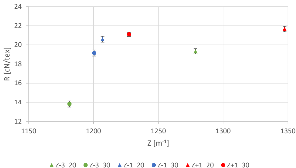
Graf 12 Vliv počtu zákrutů na poměrnou pevnost příže
