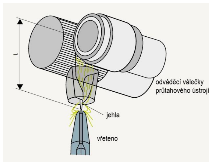
Obrázek 10 Transport vláken od průtahového ústrojí k dutému vřetenu (MVS) [3]
