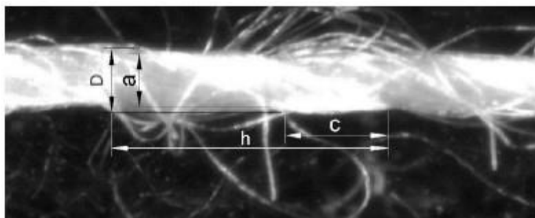
Obrázek 13 Znáornění strukturních parametrů tryskové příze dle Eldeeba [33]
