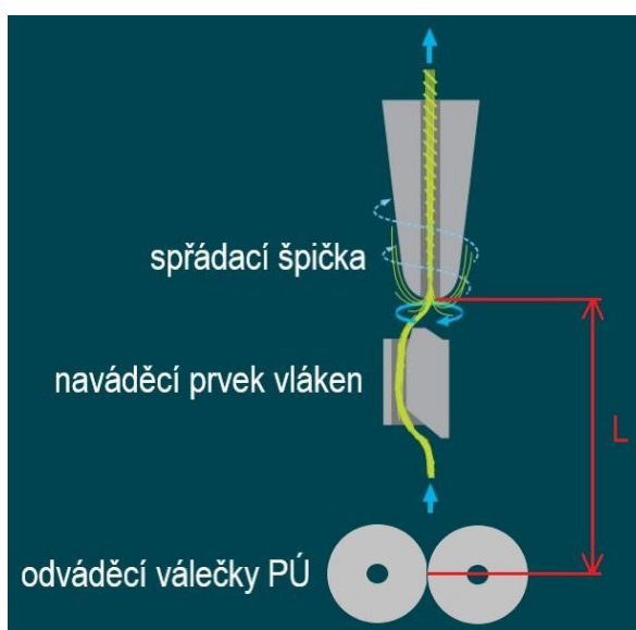
Obrázek 3 Schématické znázornění vzdálenosti L na stroji Air-Jet [4]
