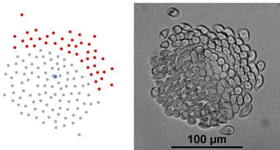
Obrázek 17 Porovnání rekonstrukce středů vláken (vlevo) s reálným snímkem řezu příze Z+1_20 (vpravo)
