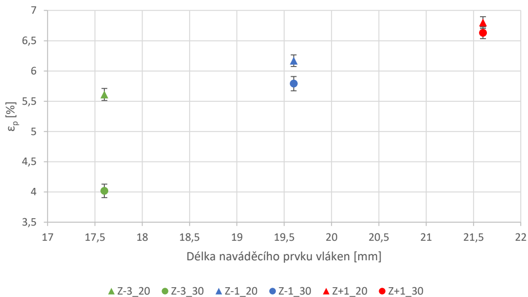
Graf 13 Vliv délky naváděcího prvku na tažnost příze
