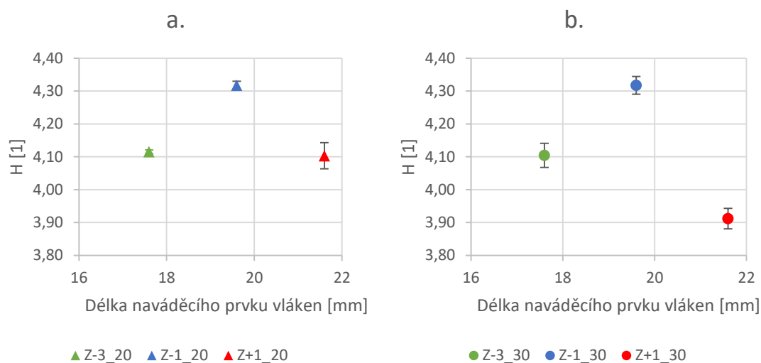
Graf 20 Vliv délky naváděcího prvku na index chlupatosti H přízí jemnosti 20 tex (a.) a 30 tex (b.)
