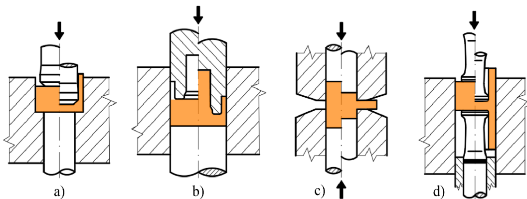
Obr. 24 Schémy hlavných spôsobov spätého pretlačovania [5]: a) späté pretlačovanie, b) uzavreté späté pretlačovanie, c) stranové pretlačovanie, d) združené pretlačovanie.
