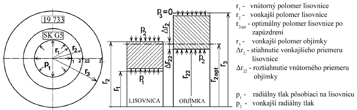
Obr. 54 Geometrický model lisovnice a objímky [49].
