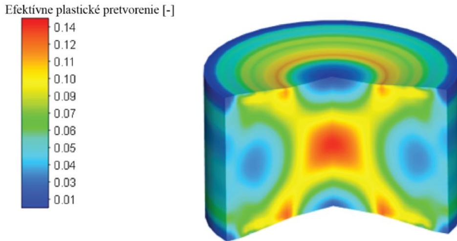
Obr. 57 Efektívne plastické pretvorenie po 1. operácií.
