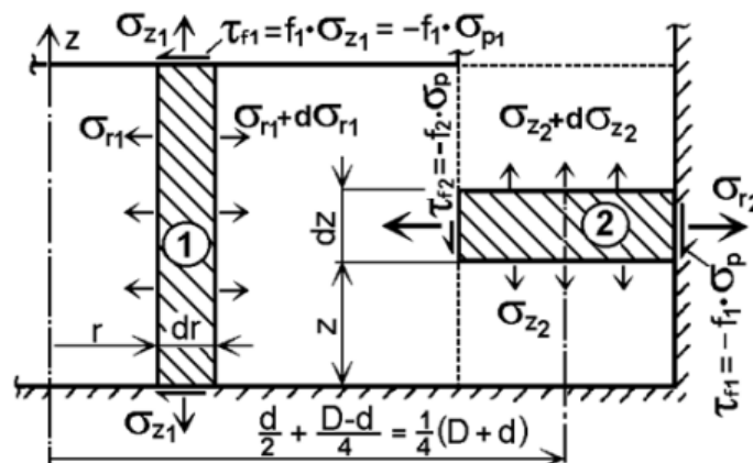
Obr. 30 Matematický model deformovanej časti prietlačku [44].
