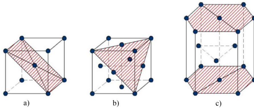
Obr. 14 Hlavné typy kryštálických mriežok a ich sklzové roviny [34]: a) BCC, b) FCC, c) HCP.
