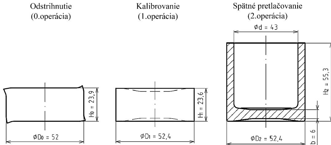
Obr. 40 Technologického postupu č.1 s vypočítanými rozmermi po jednotlivých operáciách
