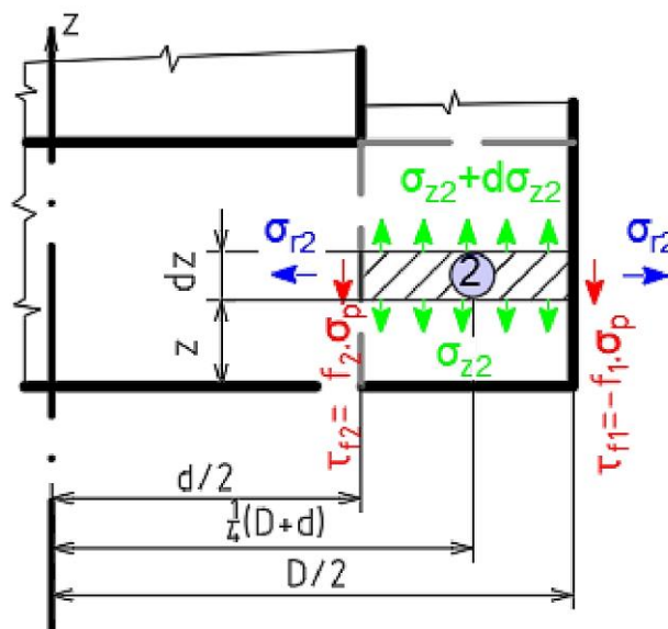
Obr. 47 Matematický model oblasti 2 [5].
