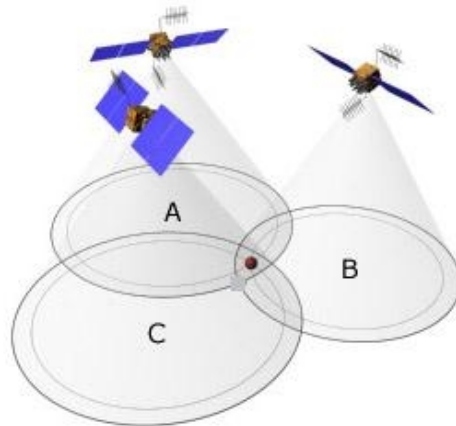
Obr. 3.6 Určení pozice v 2D rovině [15]
