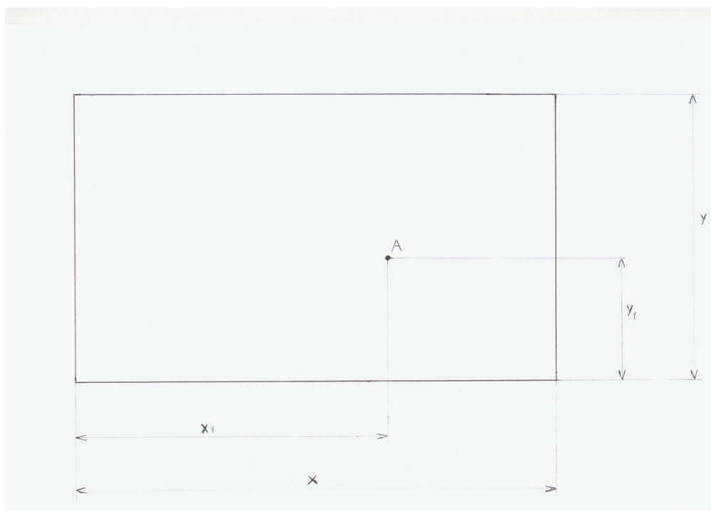
Obr. 5.1 Výpočet pozice
