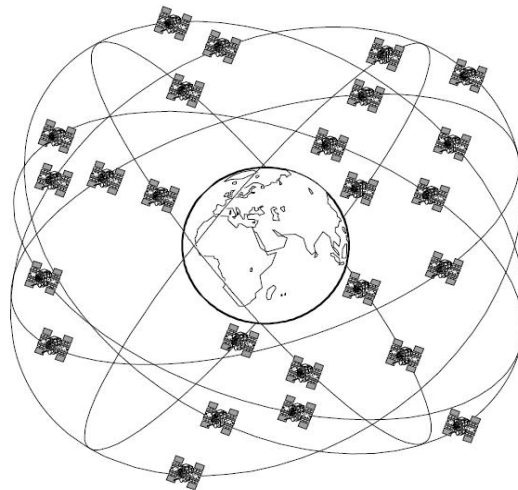
Obr. 3.1 Orbitální dráhy [2]
