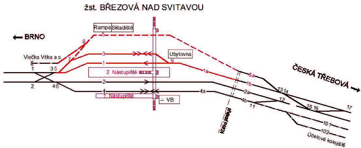
Obrázek 4: Zjednodušené schéma varianty A1
