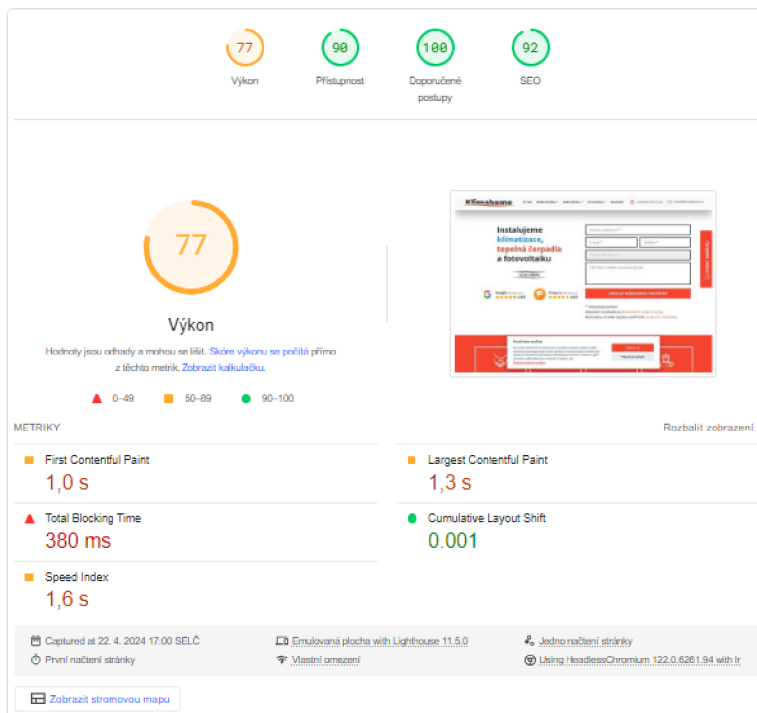
Obrázek 21 konkurence klimahome
