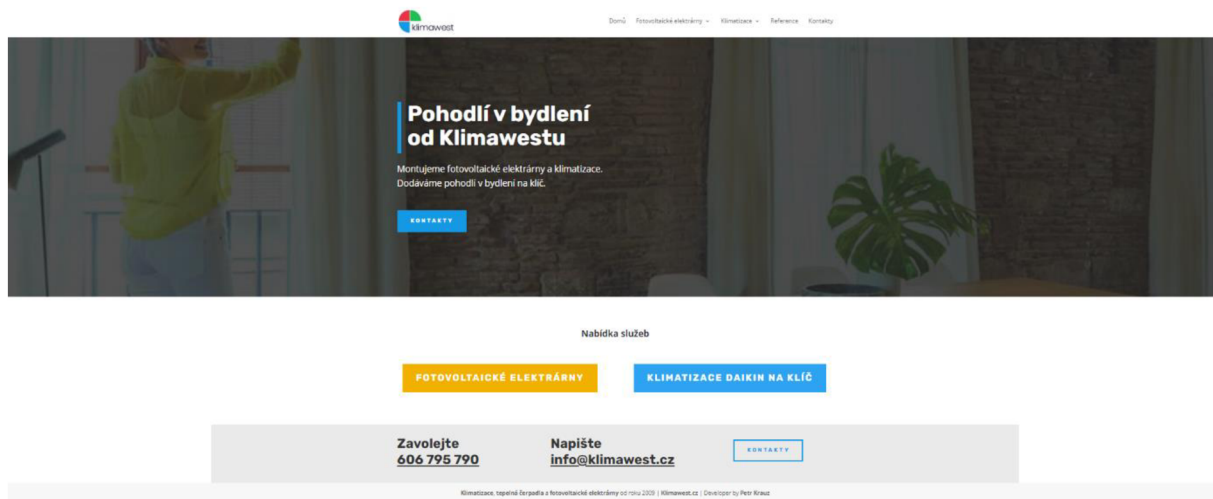
Obrázek 1 Homepage Klimawest
