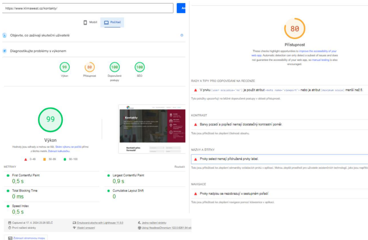
Obrázek 13 kontakty desktop
