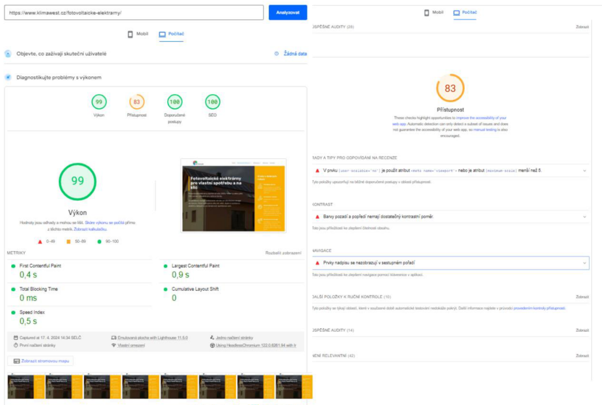
Obrázek 7 Fotovoltaika Desktop
