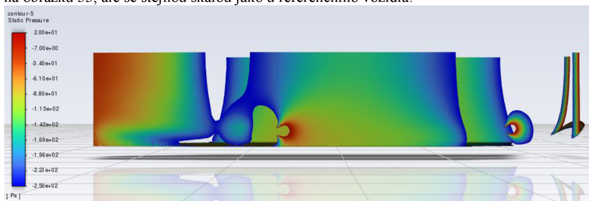
Obrázek 56: Tlak na podvozku s difuzorem (odpovídající škála tlaku)
