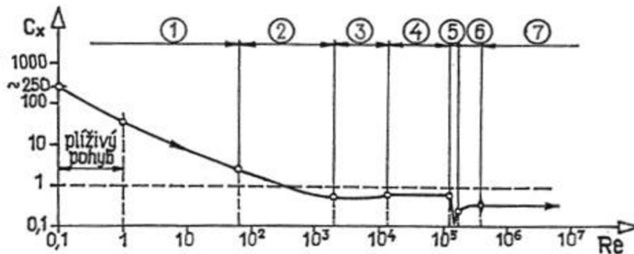
Obrázek 4: Závislost C_x na Re pro tvar koule [4]
