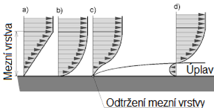
Obrázek 2: Vznik úplavu [6]
