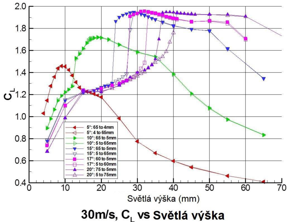
Obrázek 23: Závislost přitlaku na světlé výšce pro různé úhly, upraveno dle [36]
