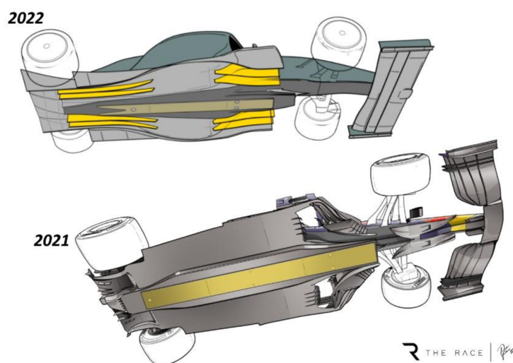
Obrázek 32: Porovnání struktury podvozků formulí ze sezón 2021 a 2022 [58]
