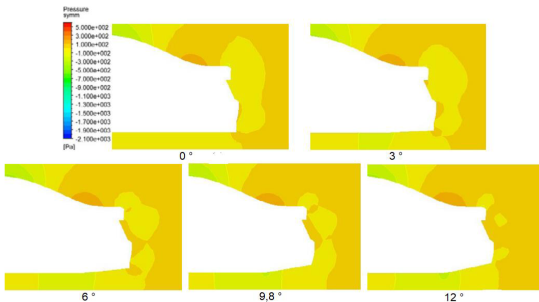
Obrázek 26: Tlakový profil v brázdě za vozidlem s různým úhlem difuzorů [37]
