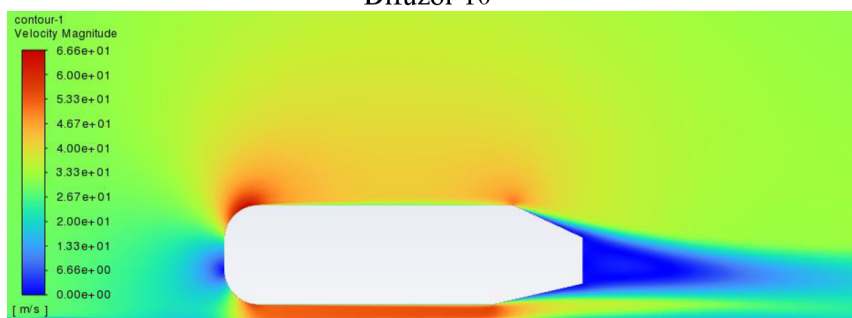
Difuzor 13 °
