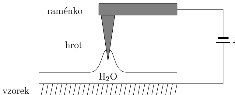
Obrázek 3.6 Schéma lokální anodické oxidace.
