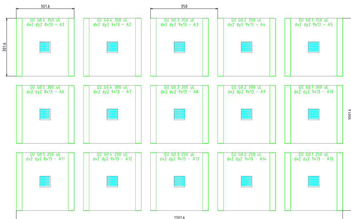
Obrázek 6.1 Rozložení polí na vzorku, D - průměr antény v \mu\text{m} , G - velikost gapu mezi anténami v \mu\text{m} , dx, dy - rozestupy mezi dvojicemi antén v \mu\text{m} , kóty jsou taktéž v \mu\text{m} .
