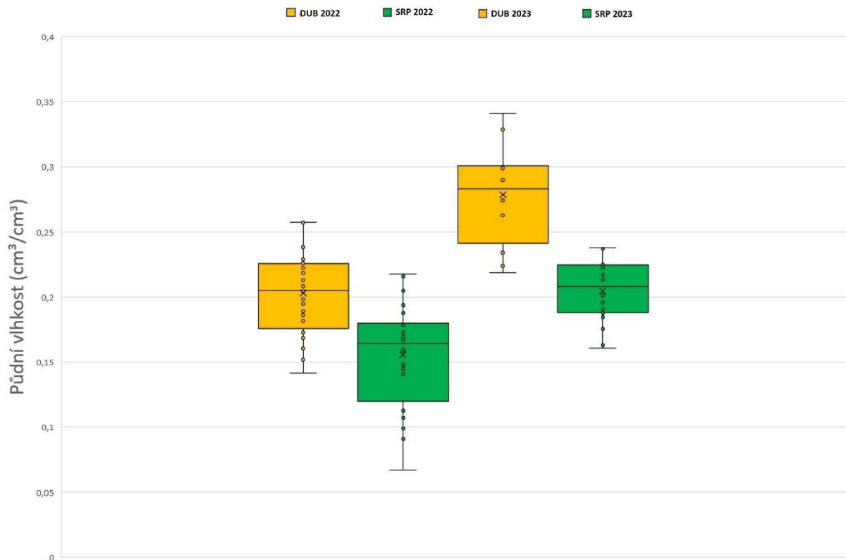
Obrázek 26.: Souhrn hodnot půdní vlhkosti pro jednotlivé sezóny ( \text{cm}^3/\text{cm}^3 ) (pořadí boxplotů: duben 2022, srpen 2022, duben 2023, srpen 2023). Křížek – průměr, vodorovná čára – medián.
