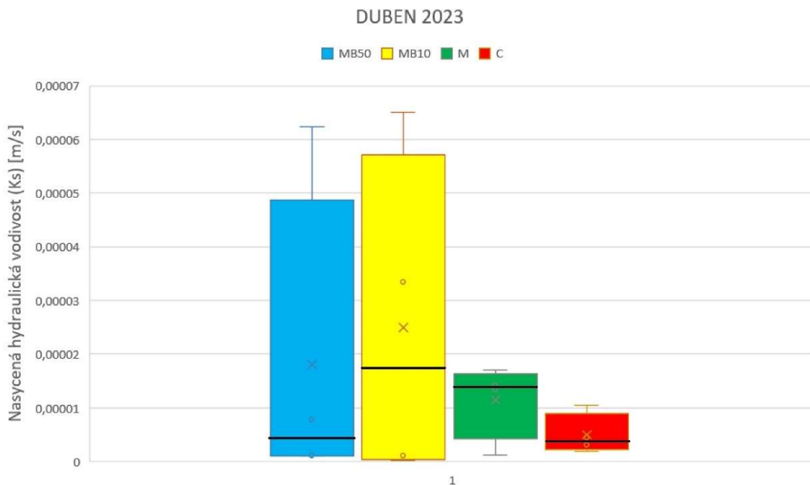
Obrázek 13.: graf naměřených hodnot nasycené hydraulické vodivosti – duben 2023, MB50 – směs hnoje a biouhlu v poměru 1:1 (modrá barva), MB10 - směs hnoje a biouhlu v poměru 1:10 (žlutá barva), M – hnůj (zelená barva), C – bez ošetření. Křížek – průměr, vodorovná čára – medián.
