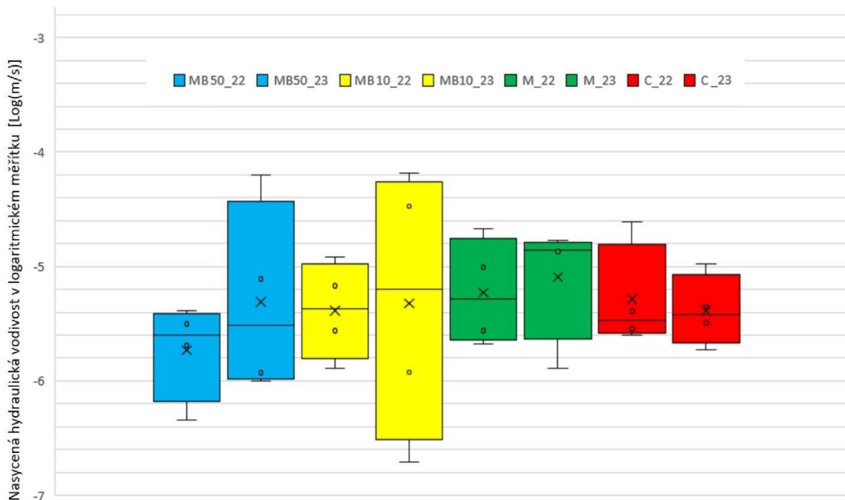
Obrázek 24.: Nasycená hydraulická vodivost v logaritmickeém měřítku [Log(m/s)] – všechny způsoby ošetření – rok 2022 (levá strana) a 2023 (pravá strana), MB50 – biouhel a hnůj v poměru 1:1 (modrá), MB10 – biouhel a hnůj v poměru 1:10 (žlutá), M – hnůj (zelená), C – bez ošetření (červená). Křížek – průměr, vodorovná čára – medián.
