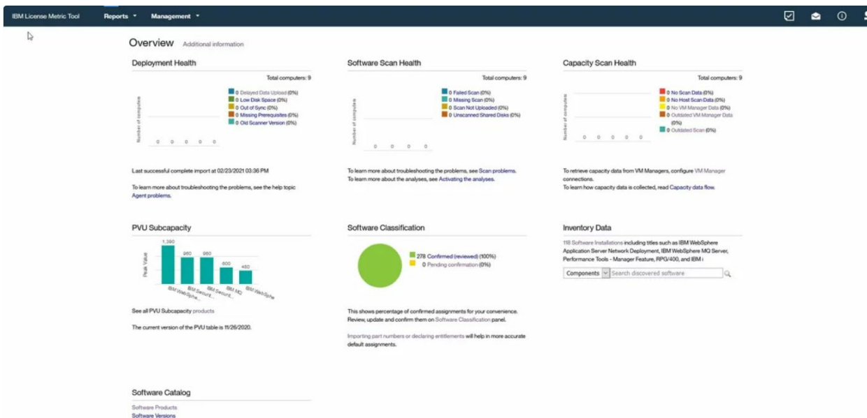
Obrázek 10 ILMT Dashboard
