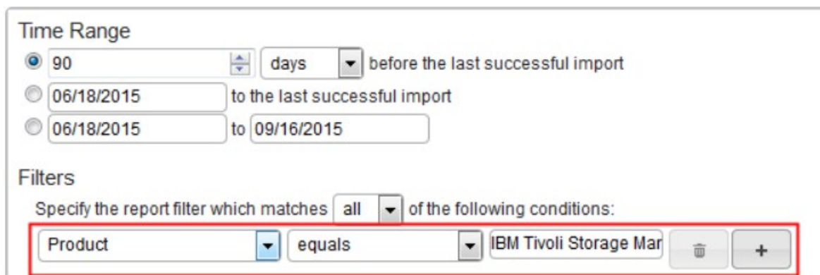
Obrázek 11 ILMT Export
