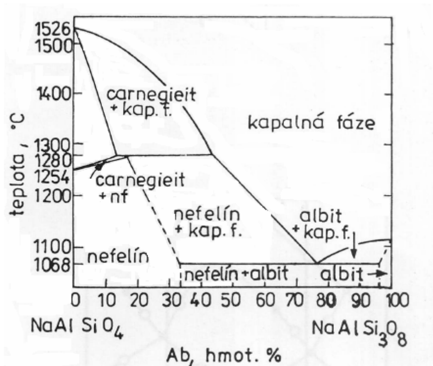
Obrázek 10: Fázový diagram systému \text{NaAlSiO}_4 (nefelin, carnegieit) - \text{NaAlSi}_3\text{O}_8 (albit) [13]
