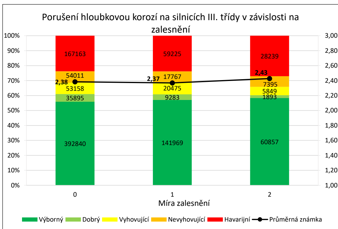
Graf 14 - Porušení hloubkovou korozí na silnicích III. třídy v závislosti na zalesnění v roce 2020
