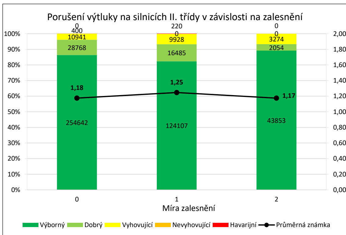
Graf 37 - Porušení výtlučky na silnicích II. třídy v závislosti na zalesnění v roce 2020
