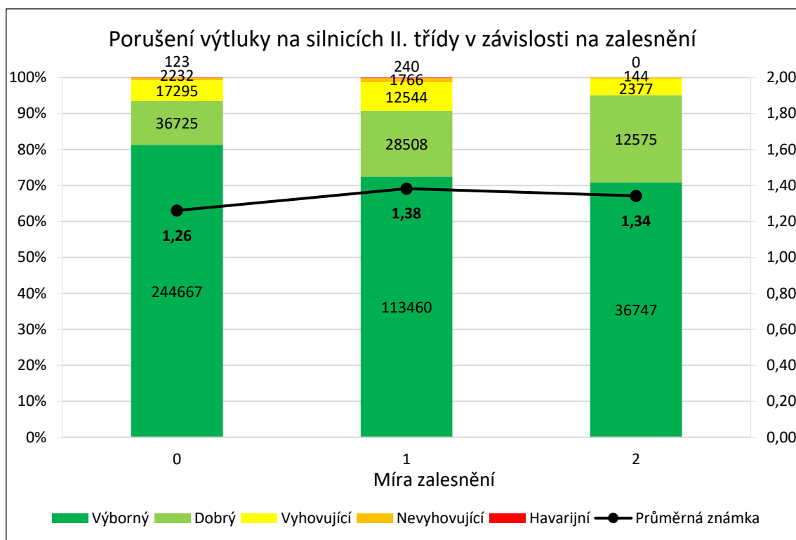
Graf 31 - Porušení výtlučky na silnicích II. třídy v závislosti na zalesnění v roce 2021
