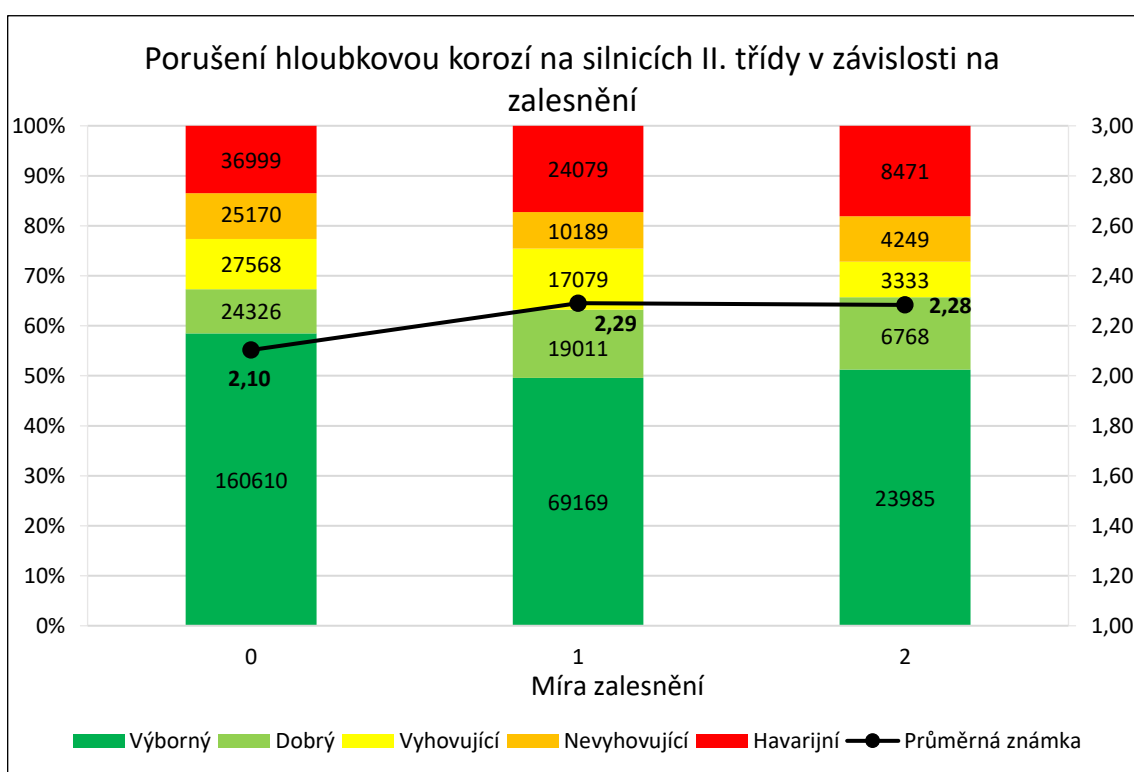
Graf 25 - Porušení hloubkovou korozi na silnicích II. třídy v závislosti na zalesnění v roce 2014
