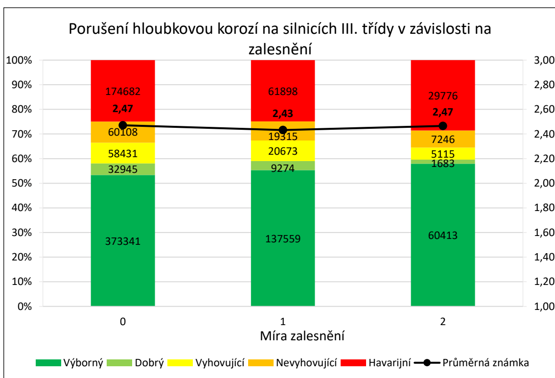
Graf 20 - Porušení hloubkovou korozí na silnicích III. třídy v závislosti na zalesnění v roce 2019
