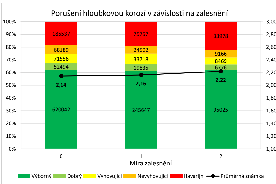
Graf 9 - Porušení hloubkovou korozi v závislosti na zalesnění v roce 2020
