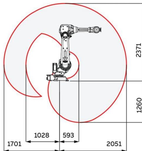
Obr. 14) Obálka dosahu príruby robota ABB IRB 4600-45/2.05 [21]
