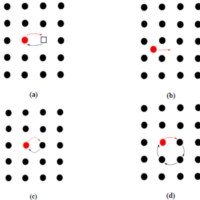
Obr. 2.1.5 Mechanismy difúze [16]
