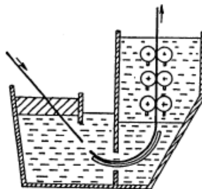
Obr. 2.6.2 Schéma žárového cínování ocelových plechů [9]
