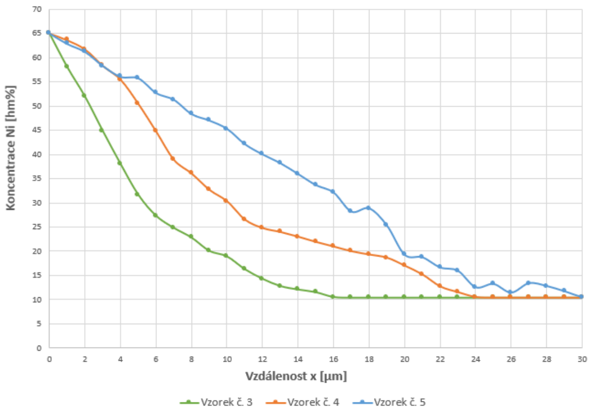
Obr. 3.4.3 Porovnání vzorků AISI 316L podle maximální teploty cyklu s výdrží 1 hodina
