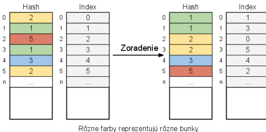
Obrázek 5.2: Zoradenie indexov podľa hash kódov v uniformnej mriežke.
