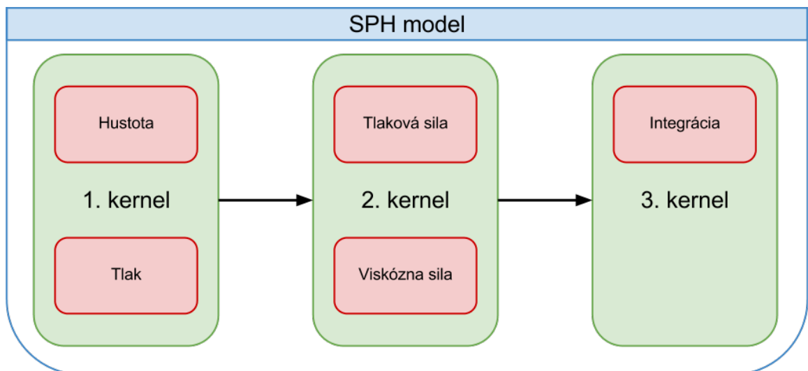
Obrázek 4.2: Navrhnutý SPH model pre GPU. Kvôli dátovým závislostiam potrebujeme tri prechody nad časticami a na každý prechod jeden GPU kernel. Každý kernel má na starosti riešiť iné úlohy.
