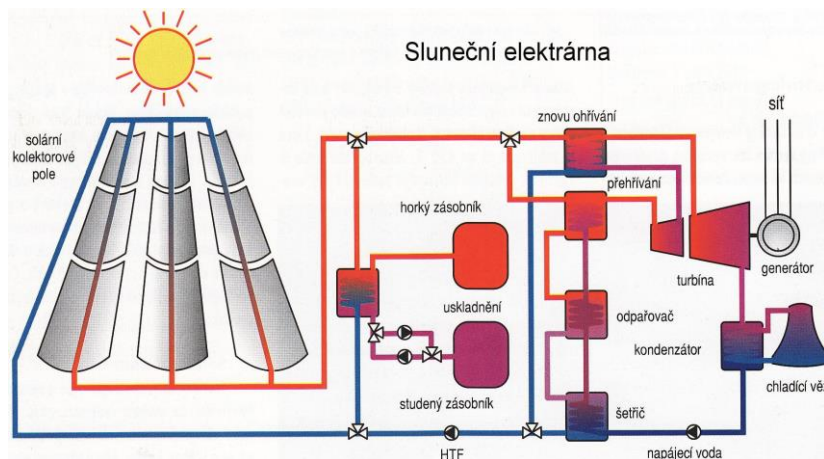
Obrázok 5.1 Solárna elektrárňa so žľabovými parabolickými kolektormi [18]
