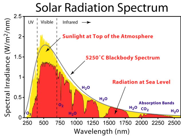
Obrázok 1.2 Slnčné spektrum [4]
