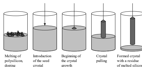
Obrázok 3.2 Výroba monokryštálu Czochralského metódou [11]
