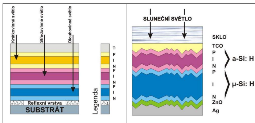
Obrázok 3.5 Trojvrstvový amorfný kremíkový článok (vľavo); tandemový mikromorfný solárny článok (vpravo) [14]
