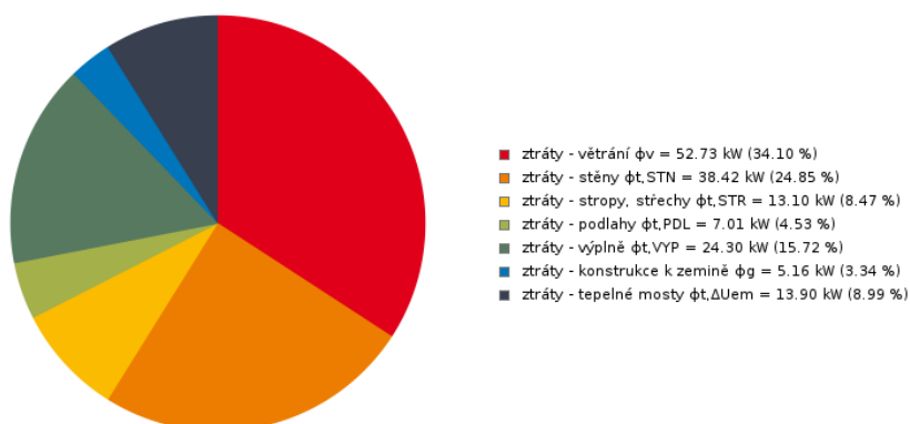
Graf 10.1 Tepelné straty prestupom konštrukcií a vetraním
