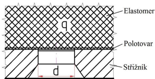
Obr. 2.2 Prostřihování otvoru
