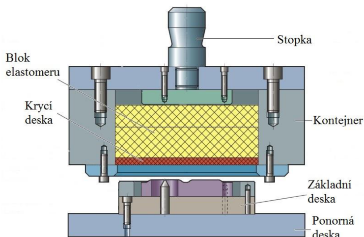
Obr. 2.4 Nástroj pro kombinaci stříhání a tažení [5]
