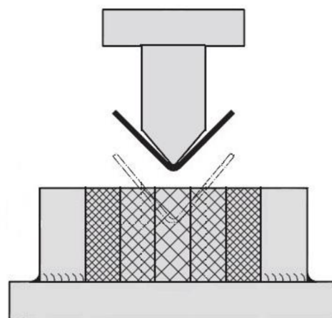
Obr. 1.1 Otevřený nástroj [5]
