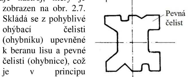
Obr. 2.7 Konvenční ohýbadlo [2]
