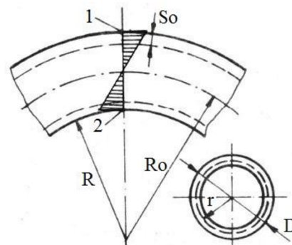
Obr. 2.9 Geometrie ohybu trubky a průběh přetvoření v osovém směru [2]
