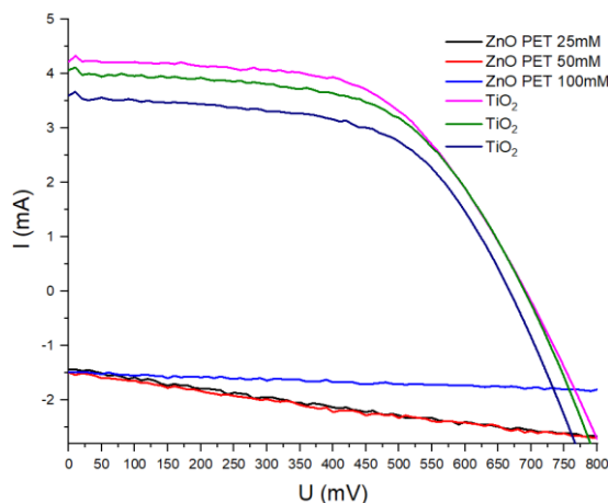
Graf 13: Proudovo-napěťová charakteristika DSSC založených na ZnO pracovních elektrodách připravených na ITO substrátech.
