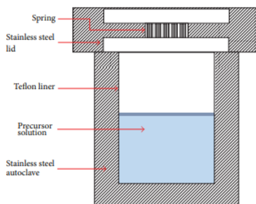
Obrázek 23: Schéma autoklávu používaného při solvotermální a hydrotermální syntéze [57].
