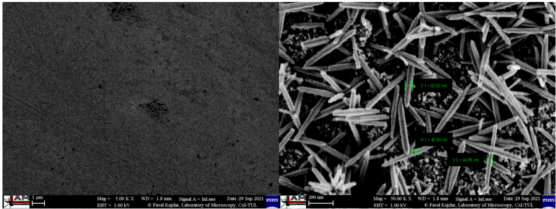
Obrázek 45: SEM snímky nanotyčinek připravených pomocí klasické syntézy na ITO substrátu.
