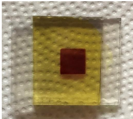
Obrázek 38: DSSC článek připravený z \text{TiO}_2 elektrody.
