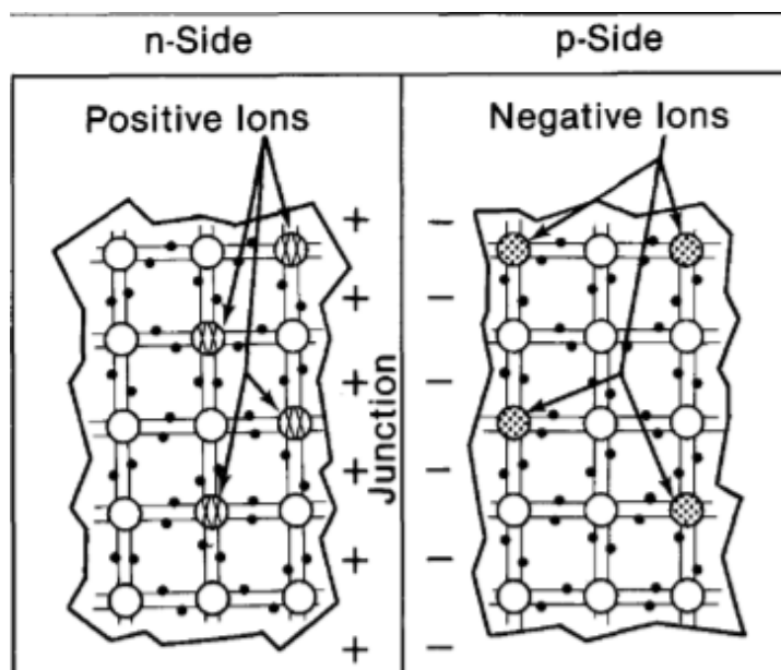
Obrázek 4: PN přechod [15].
