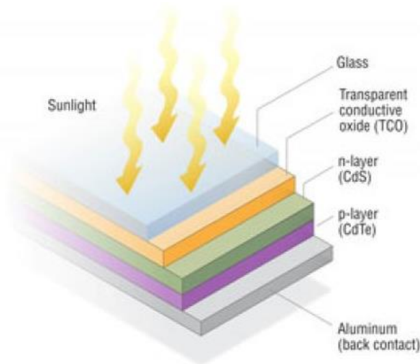
Obrázek 14: Příklad CdTe článku [45].
