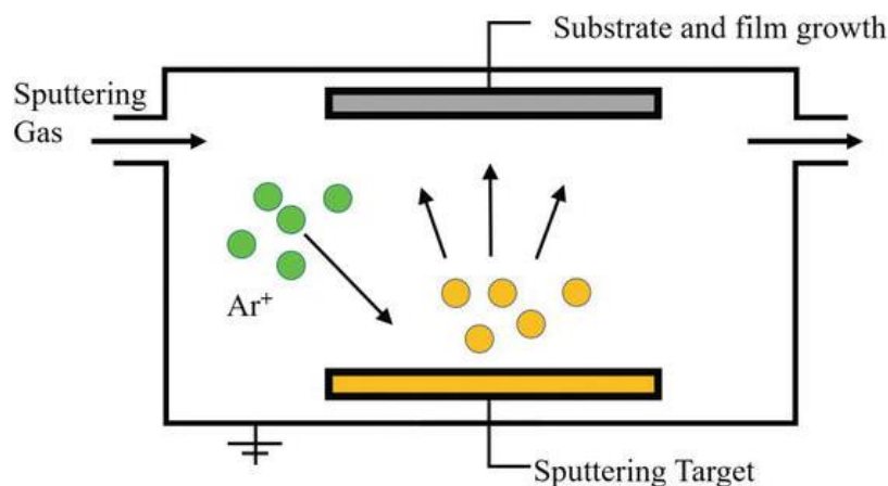
Obrázek 22: Schéma naprašování [62].
