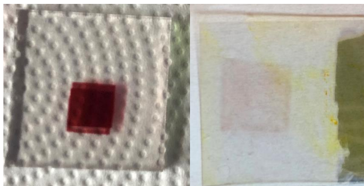
Obrázek 47: Vzorek \text{TiO}_2 (vlevo) a ZnO (vpravo) po barvení. Vzorek ZnO už je po reakci s elektrolytem.
