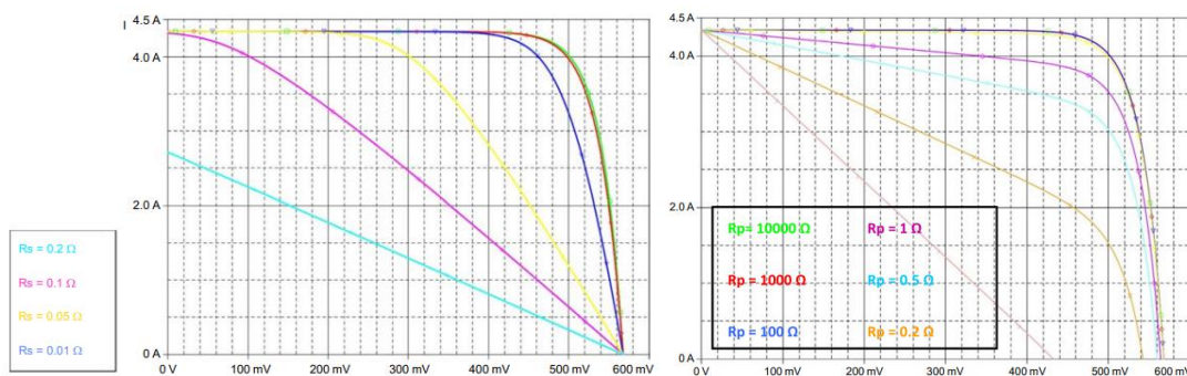
Graf 6: Vliv sériového (A) a paralelního (B) odporu na proudovo-napěťovou charakteristiku solárního článku [32].
