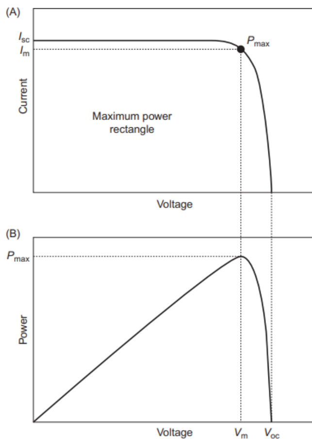
Graf 5: Proudovo-napěťová charakteristika ideálního solárního článku (A) a výkon produkovaný článkem (B) [33].
