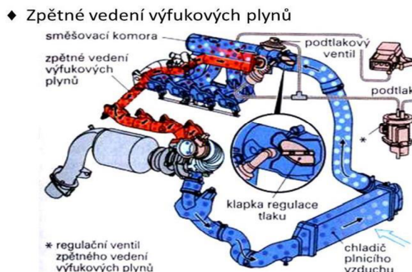
Obrázek 1.4 - Zpětné vedení výfukových plynů (NLRacing.cz, 2017)
