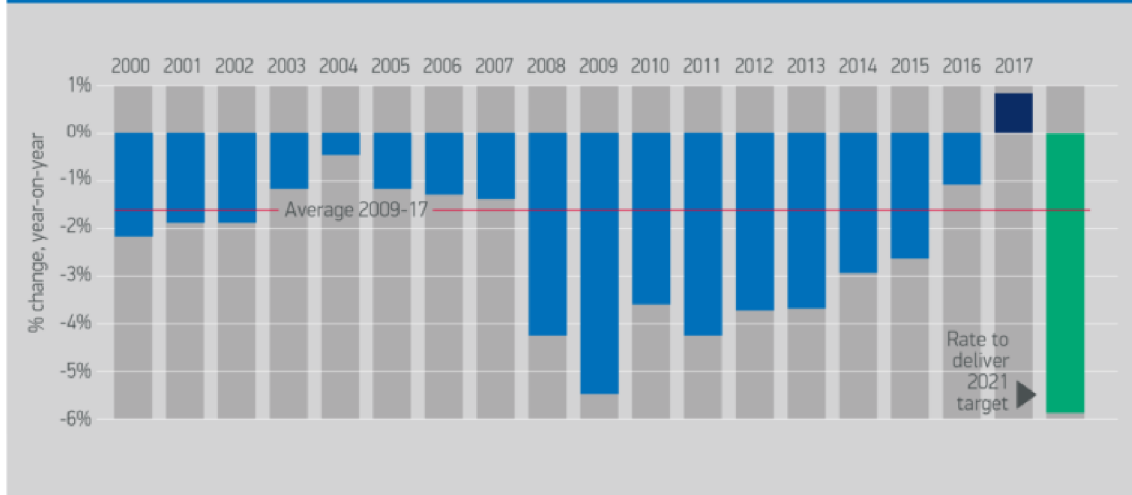
Obrázek 4.2 - Změna ročních emisí CO 2 u nových automobilů od roku 2000 (smtt.co.uk, 2018)
