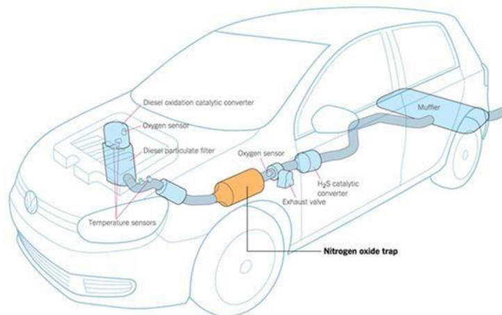
Obrázek 3.2 - Emisní soustava Volkswagenu (thetstreet.com, 2017)
