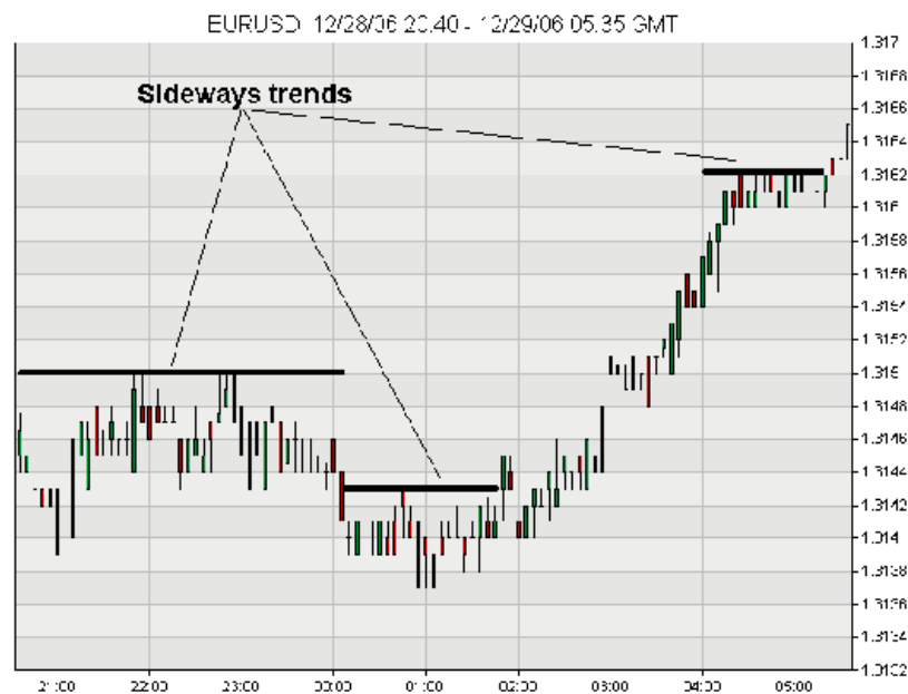
Obr. 2.3 postranný trend [19]
