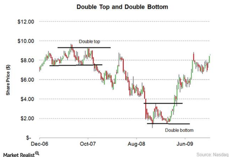
Obr. 2.11 Dvojité vrchol [21]
