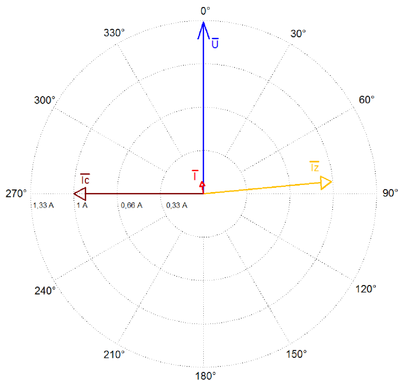
Obrázek 4-7 Fázorový diagram pro 4-6
