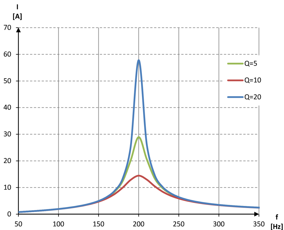
Obrázek 2-4 Závislost proudu filtru na kmitočtu
