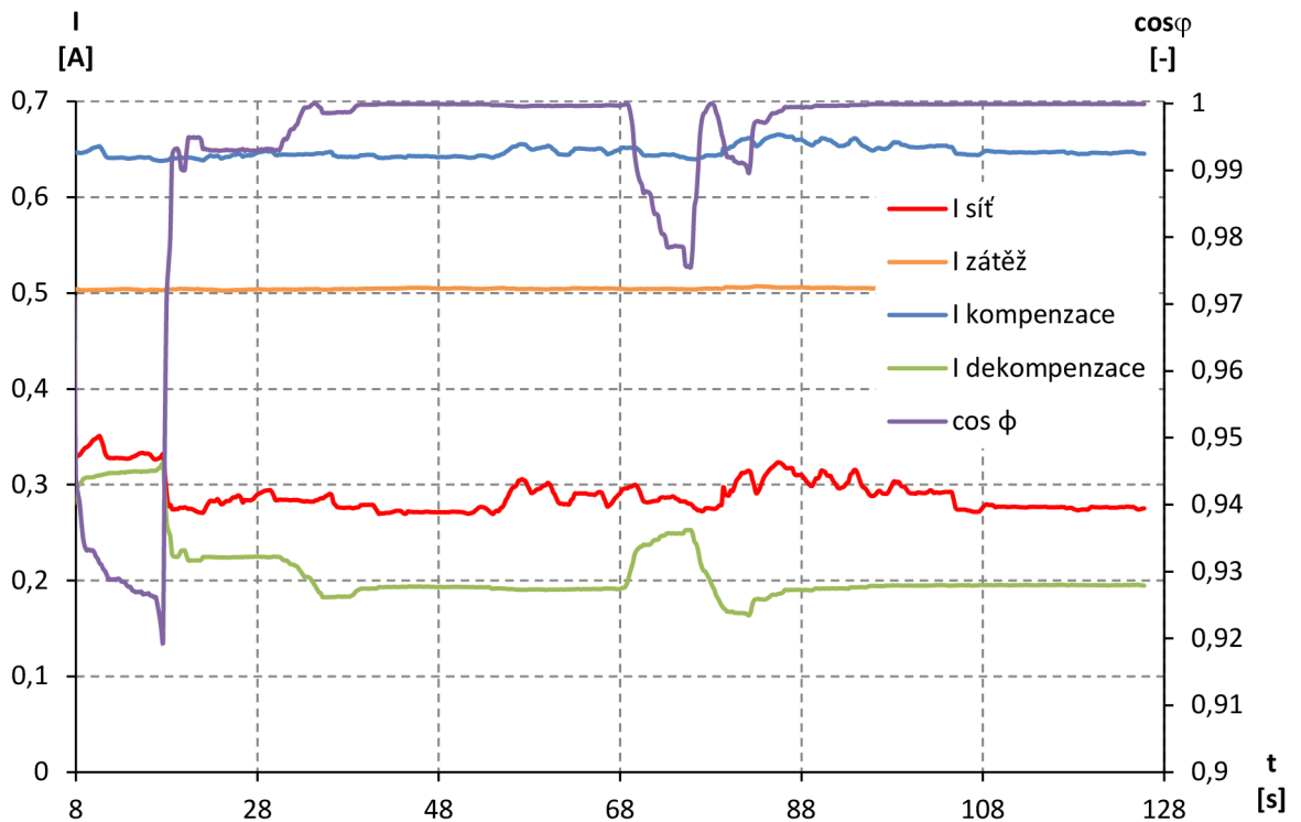
Obrázek 6-12 Řízení protékajícího proudu přes dekompenzační tlumivku
