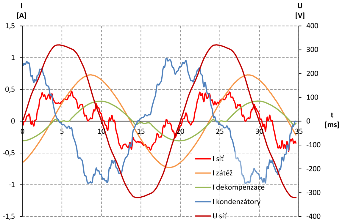
Obrázek 6-13 Časový průběh při zapnuté dekompenzaci
