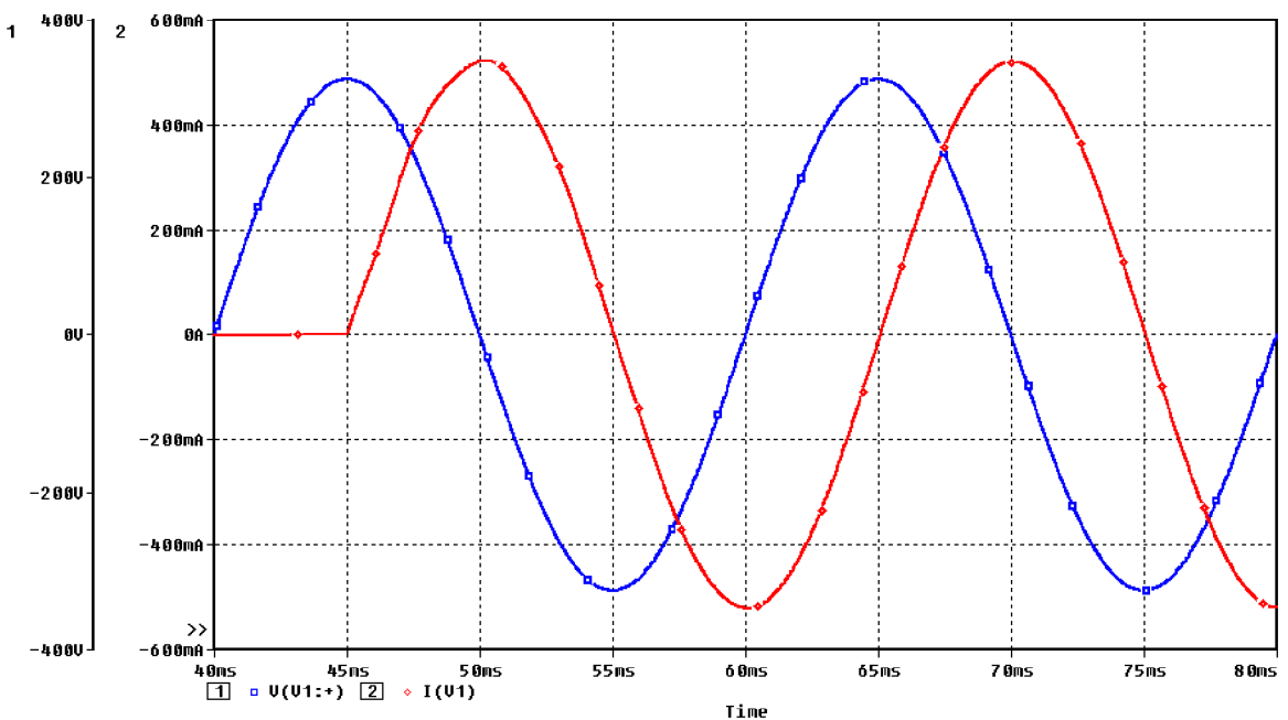
Obrázek 4-4 Připojení nabitého kondenzátoru při průchodu napětí amplitudou
