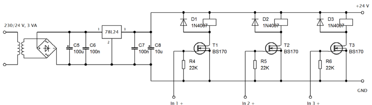
Obrázek 5-2 Schéma zapojení ovládací části modelu vedení
