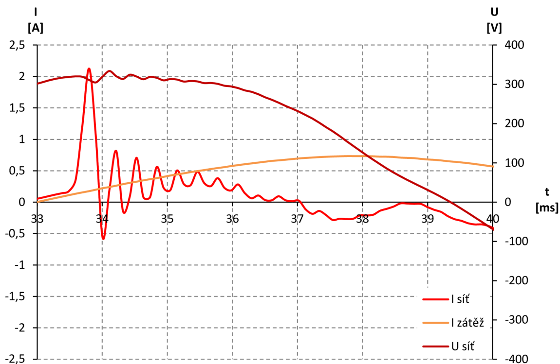
Obrázek 6-10 Detail přechodného děje přiřipnutí kondenzátoru
