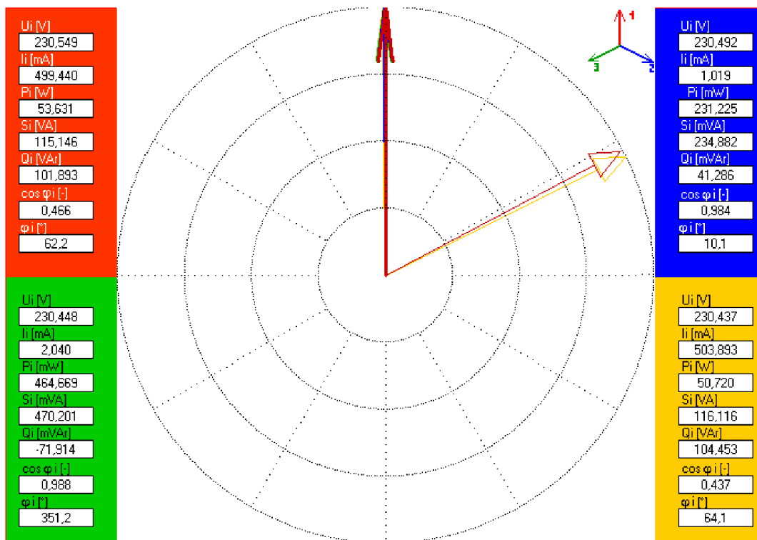
Obrázek 6-4 Fázorový diagram pro 6-3
