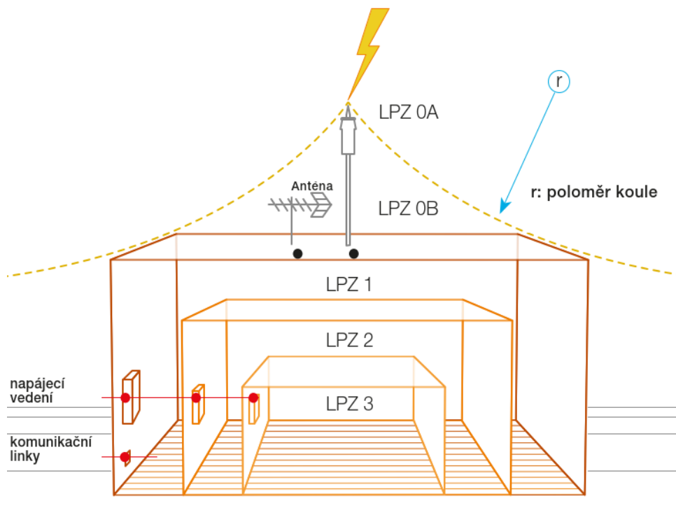
Obr. 6.4: Zóny LPZ [22].
