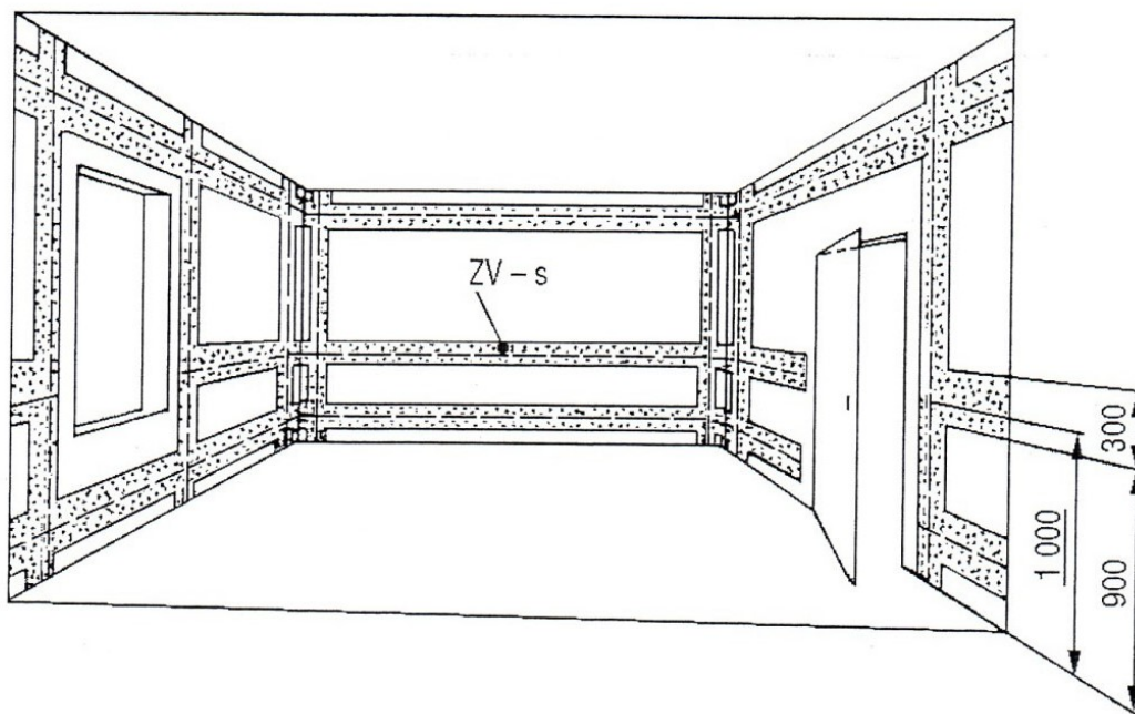
Obr. 7.2: Zóny pro ukládání elektrického vedení v kuchyni, pracovně [24].
