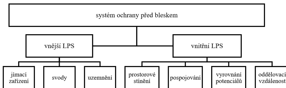
Obr. 6.1: Systém ochrany před bleskem [16].
