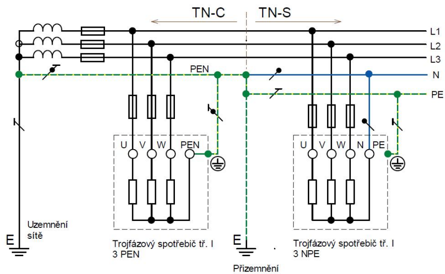
Obr. 2.5: Síť TN-C-S [5].
