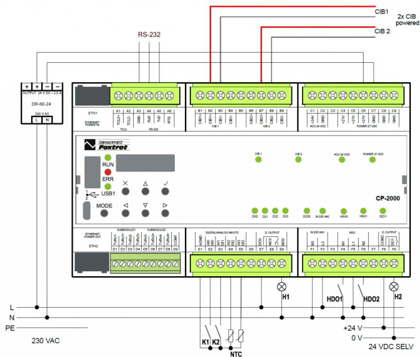
Obr. 9.5: Schéma zapojení CP-2000 [32].
