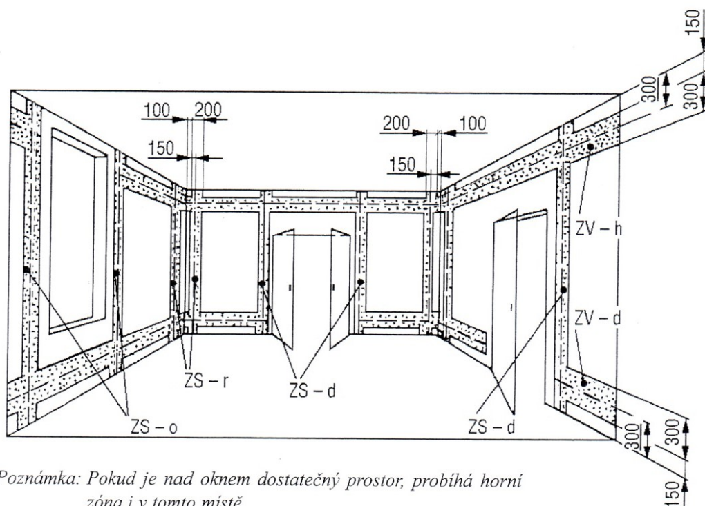
Obr. 7.1: Zóny pro ukládání elektrického vedení v pokojích [24].
