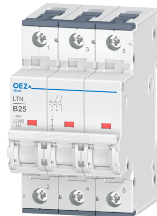
Obr. 5.4: Třípolový jistič [13].
