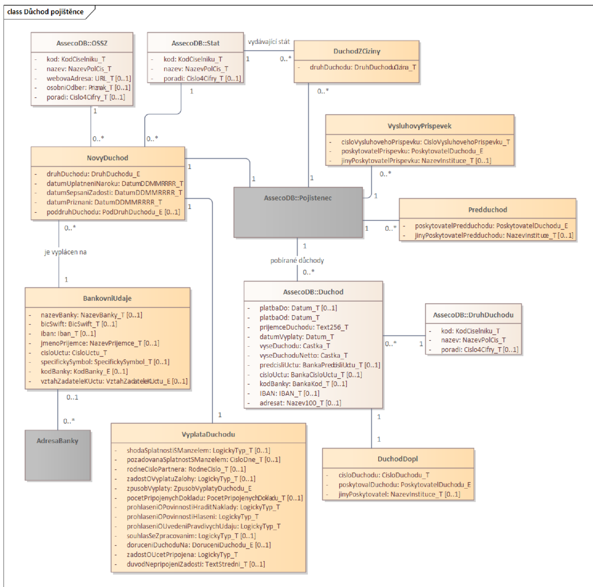
Obrázek č. 27: KDM Důchod pojištěnce
