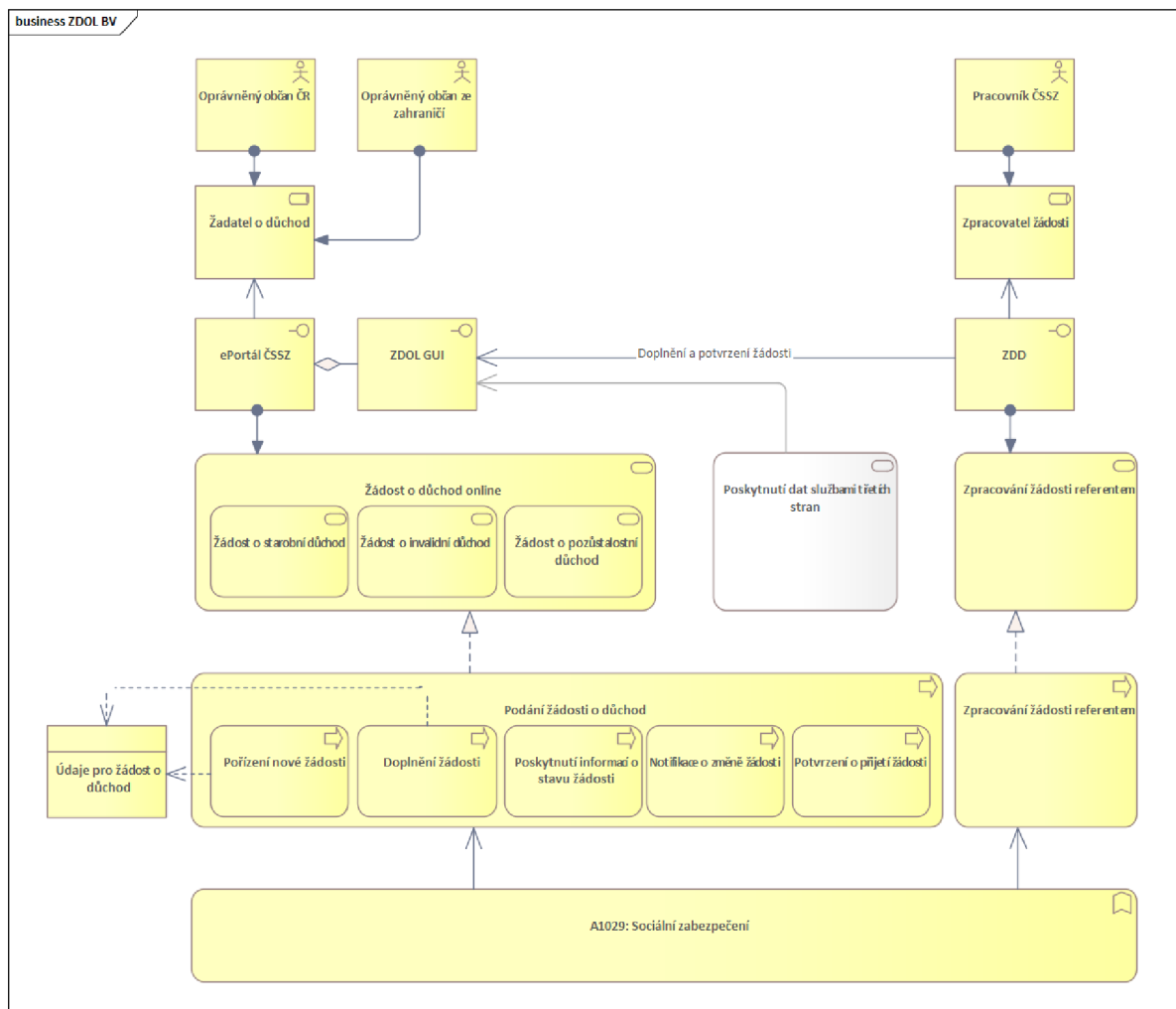
Obrázek č. 21: Business architektura aplikace ZDOL
