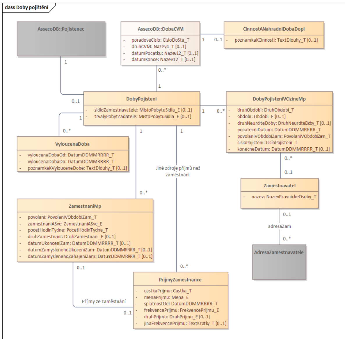
Obrázek č. 25: KDM Doby pojištění
