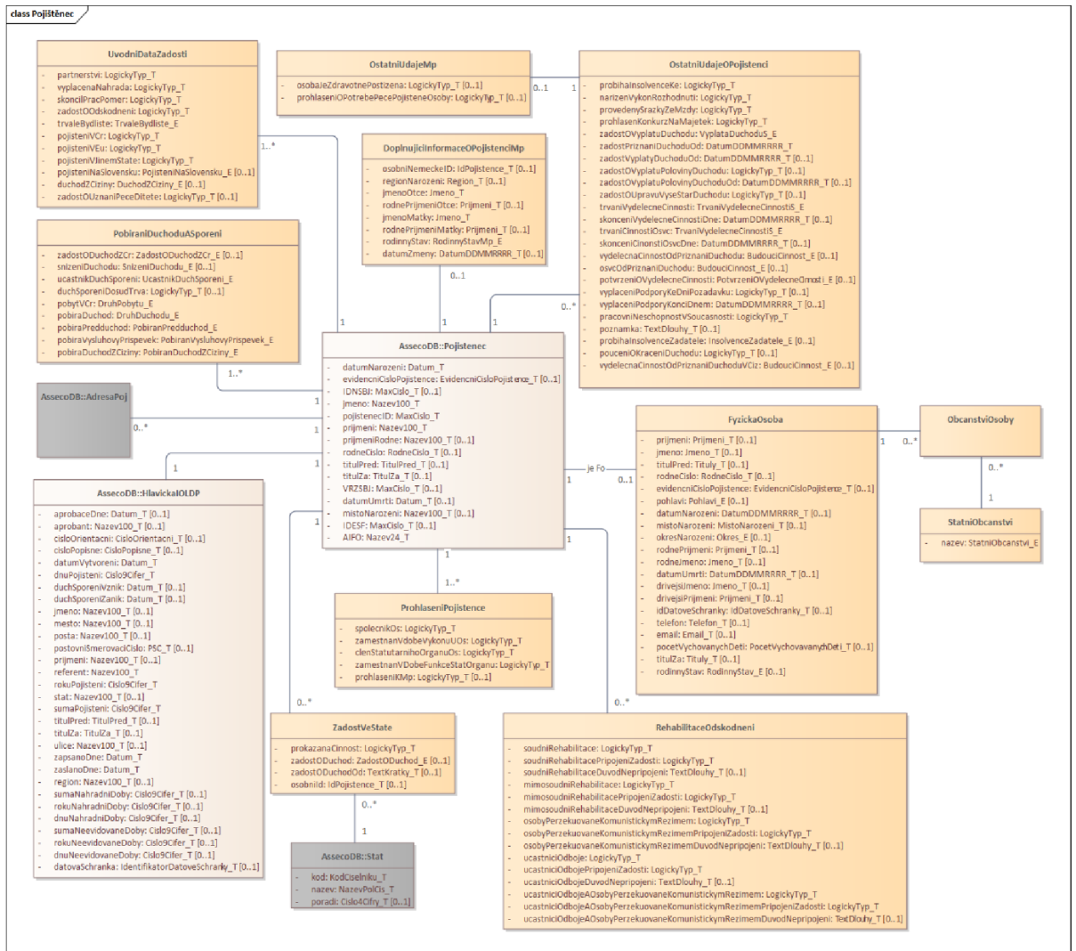
Obrázek č. 28: KDM Pojištěnec
