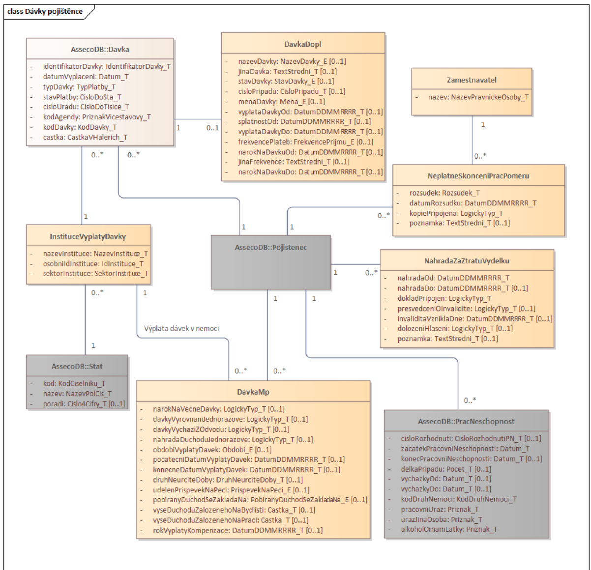
Obrázek č. 24: KDM Dávky pojištění
