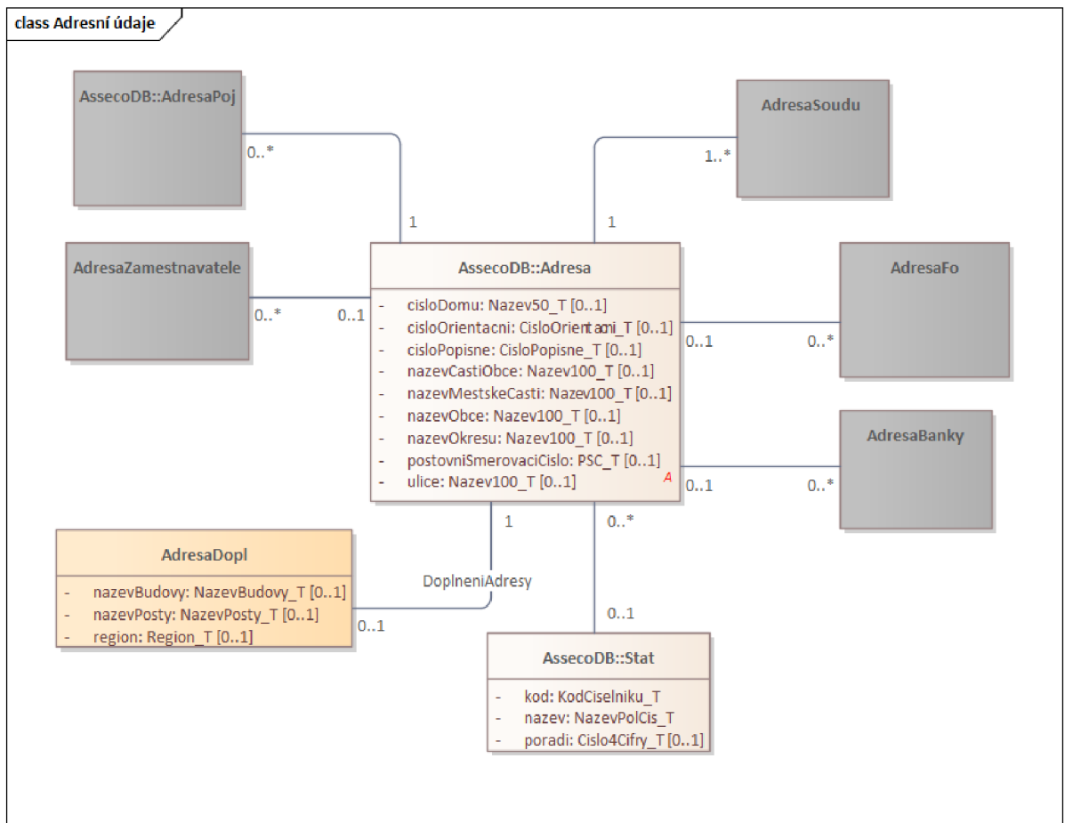
Obrázek č. 23: KDM Adresní údaje
