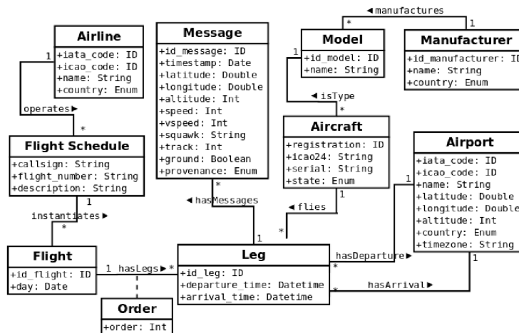
Obrázek č. 4: Ukázka konceptuálního datového modelu
