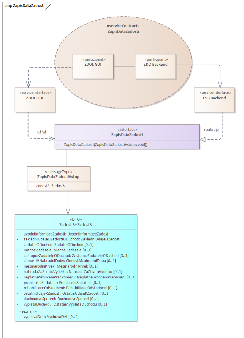
Obrázek č. 32: Služba pro zápis dat v ZDD
