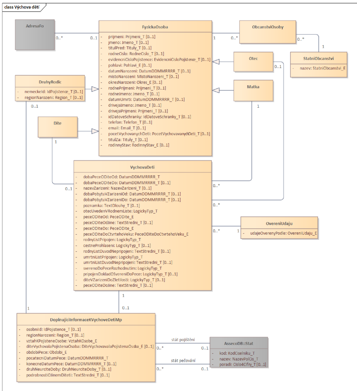
Obrázek č. 29: KDM Výchova dětí
