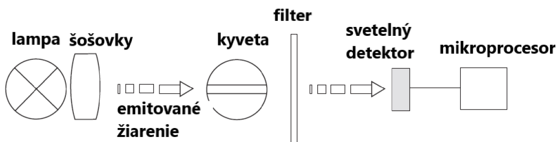
Obrázok 6: Princíp fotometru [14]
