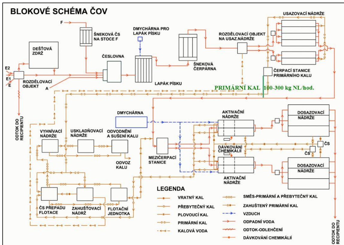
Obr. 3.3 Blokové schéma ČOV Brno – Modřice [18]
