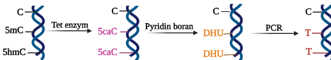
Obr. 9: Přehled reakcí metody TET asistovaného pyridin boranového sekvenování (TAPS). V první reakci je 5-metylcytozin (5mC) a 5-hydroxymetylcytozin (5hmC) oxidován Tet enzymem na 5-karboxycytozin (5caC). 5caC je redukován pyridin boranem na dihydrouracil (DHU). DHU je PCR reakcí čten jako thymin. Vytvořeno v Biorender.com dle Liu et al. , 2019.
