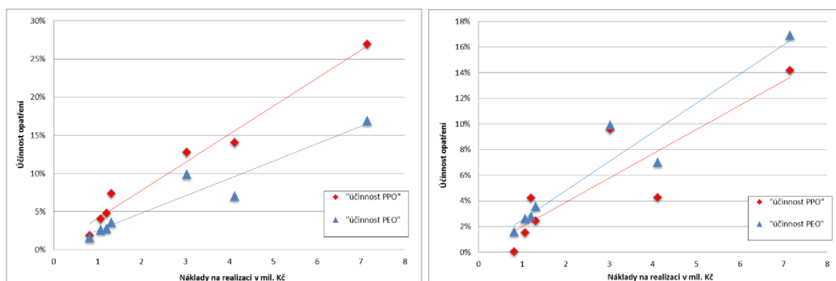
Obr. 14 Závislost nákladů na realizaci průleहů a jejich protipovodňové a protierozní účinnosti pro povodí Němčického potoka pro Q 10 vlevo a Q 100 vpravo. Znáznorněny jsou taktěž lineární regresní závislosti.
