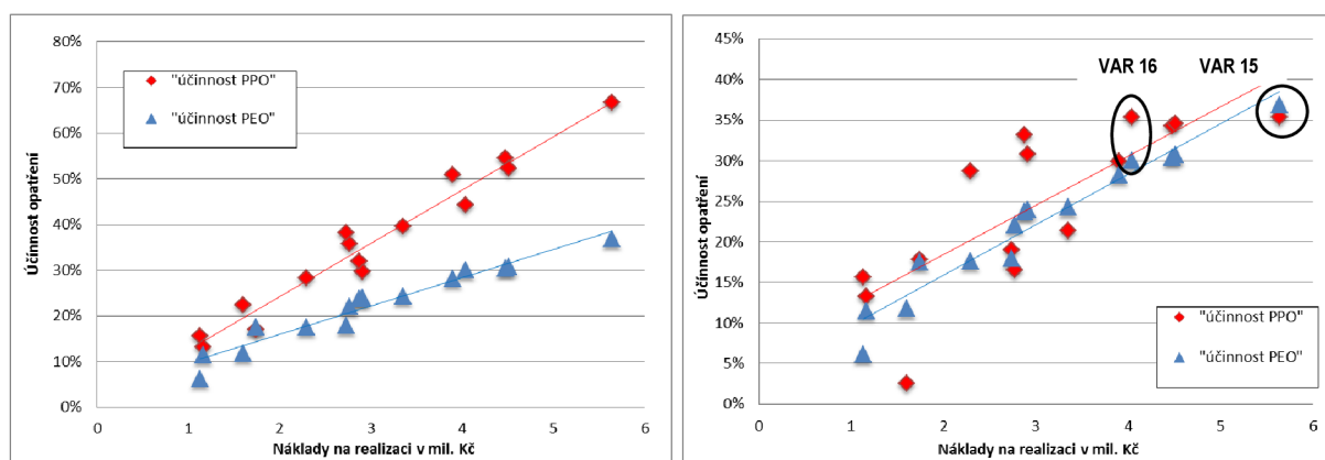
Obr. 13 Závislost nákladů na realizaci průleहů a jejich protipovodňové a protierozní účinnosti pro povodí Starovického potoka pro Q_{10} vlevo a Q_{100} vpravo. Znázorněny jsou také lineární regresní závislosti.
