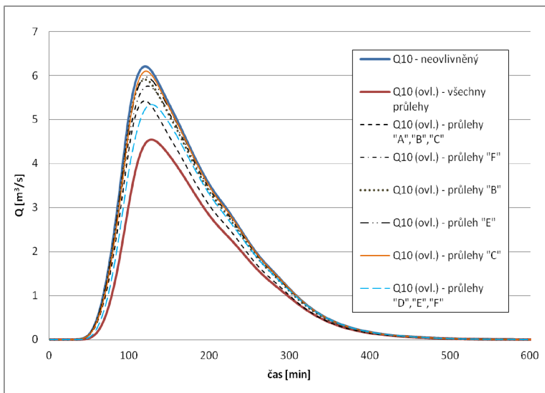
Obr. 8 Ovlivnění průtoku v závěrovém profilu v případě variant uvedených v tabulce 9
