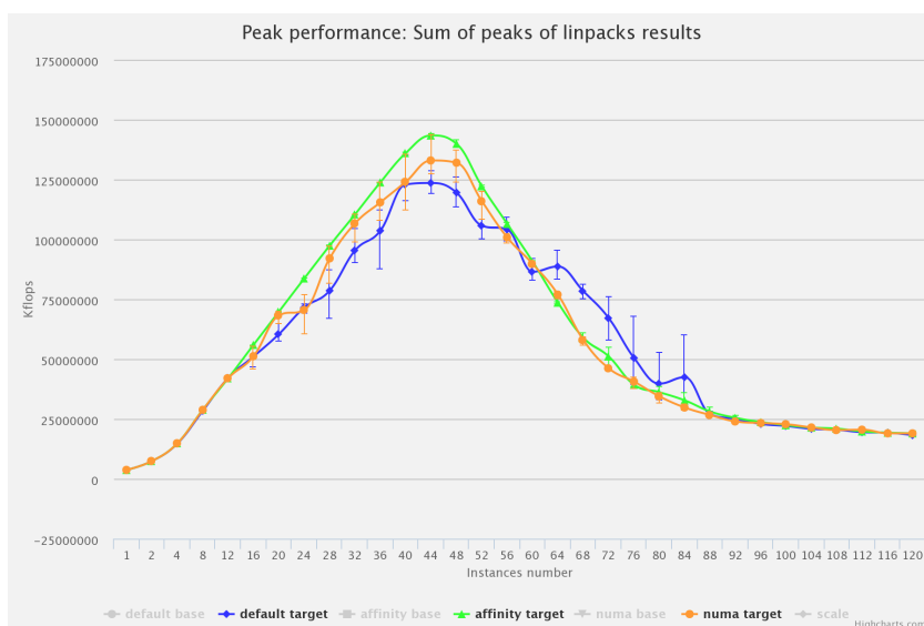
Obrázek 14: Výsledky linqpacku na jádru 3.10.0
