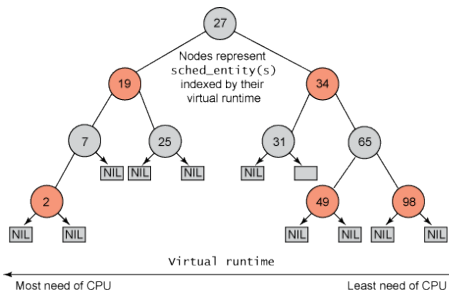
Obrázek 4: RB strom úloh setříděný podle hodnot vruntime, zdroj [TJONES]
