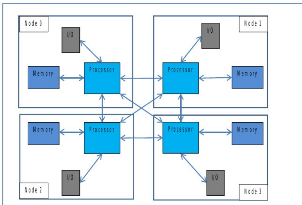
Obrázek 8: Jednoduchá NUMA topologie, zdroj [RRIEL]
