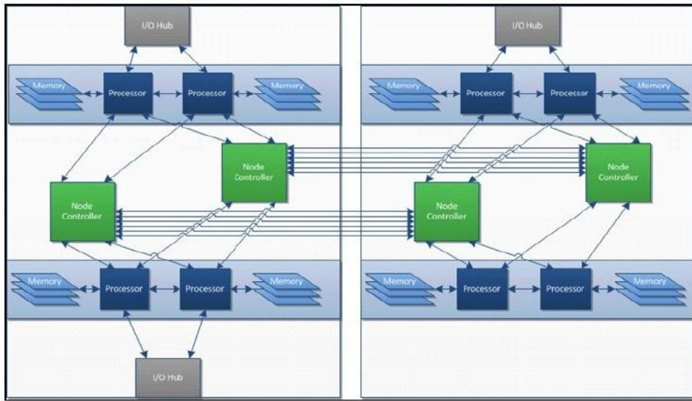
Obrázek 9: Systém se složitější NUMA topologií, zdroj [RRIEL]
