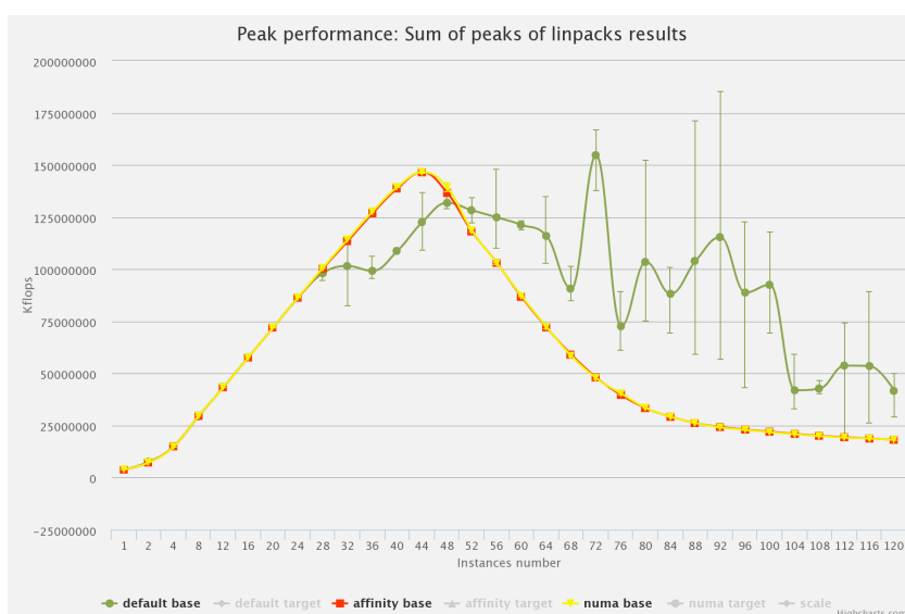
Obrázek 13: Výsledky linqpacku na jádru 2.6.32
