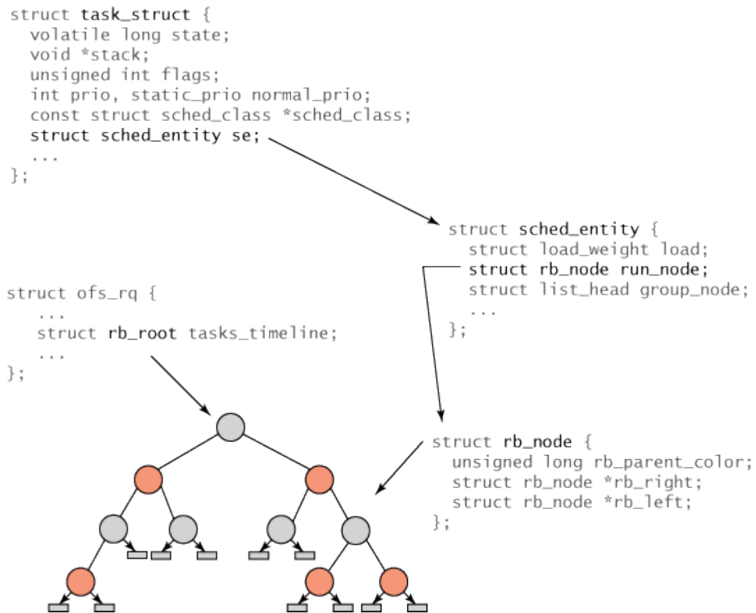
Obrázek 6: Schéma složení struktur plánovače, zdroj [TJONES]
