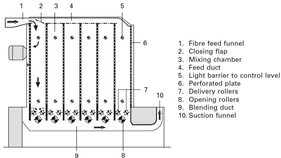
Obrázek 4: Schéma míšící komory (Russell 2007)
