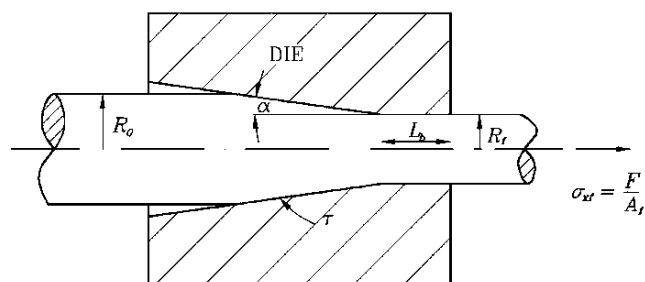
Obrázek 17: Geometrie procesu tažení. R_0 - poloměr na vstupu do matrice, R_f - poloměr na výstupu z matrice, \alpha - úhel matricí, L_b - nosná délka, \sigma_{xf} - tahové napětí (Panteghini a Genna 2010)
