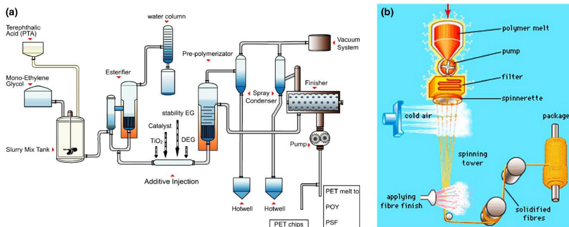
Obrázek 2: Schéma esterifikace a zvlákňování PET (Puli et al. 2021)
