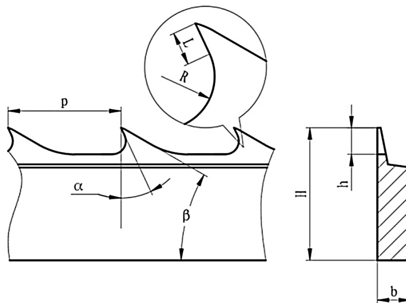
Obrázek 8: Schéma pilkového povlaku. L - rovina zubu, R - spodní oblouk, p - rozteč zubů, \alpha - pracovní úhel, H - celková hloubka, b - celková šířka, h - hloubka zubu (Gu et al. 2021)
