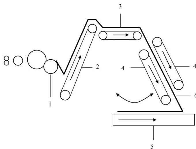
Obrázek 9: Schéma vertikálního kladečího zařízení. 1 - snímací válec, 2 - příváděcí pás, 3 - pavučina, 4 - dvojice výkyvných kladečích pásů, 5 - příváděcí pás k vypichovacímu stroji, 6 - pavučina (Kuo et al. 2007)
