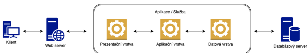
Obrázek 3.11 - Monolit schéma [22]
