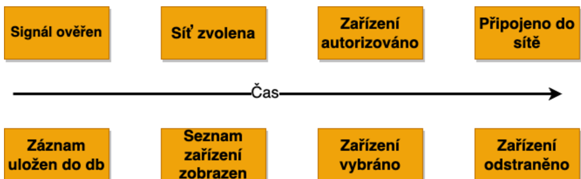
Obrázek 4.4 - Doménové události
