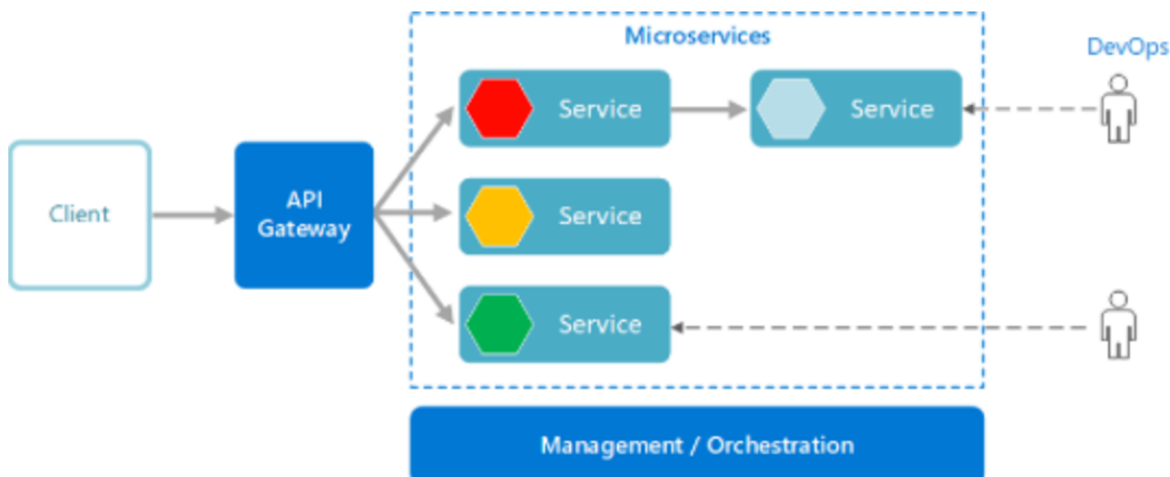
Obrázek 3.12 - Koncept Mikroslužeb [23]
