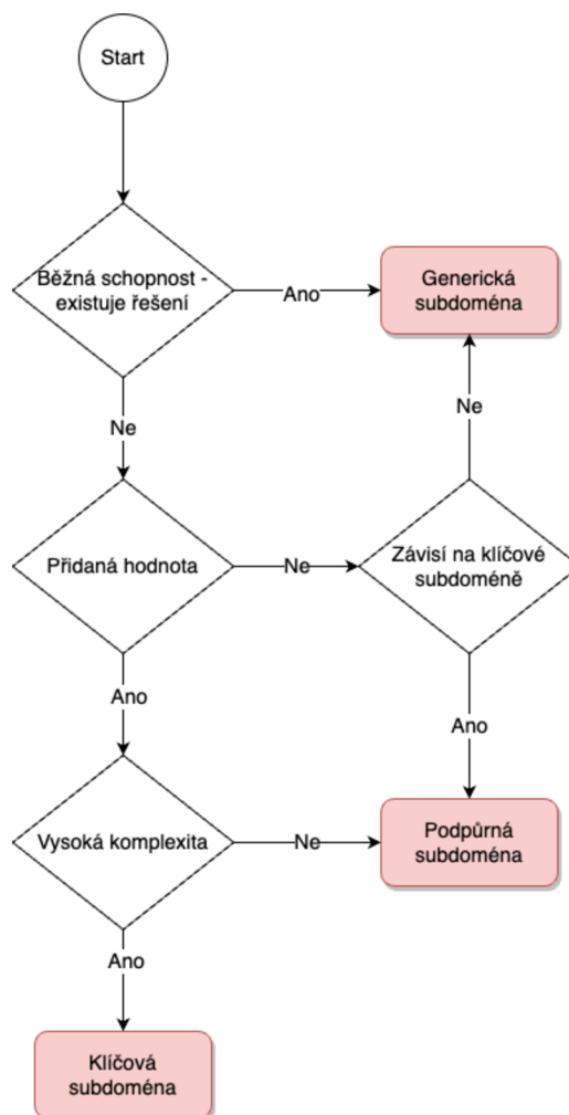
Obrázek 3.14 – Subdomény [27]
