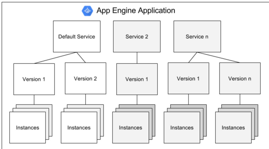
Obrázek 3.8 - Struktura App Engine [17]
