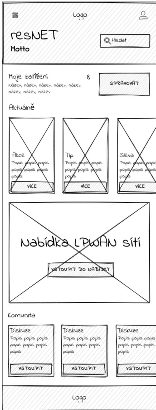
Obrázek 4.18 - WireFrame HomePage
