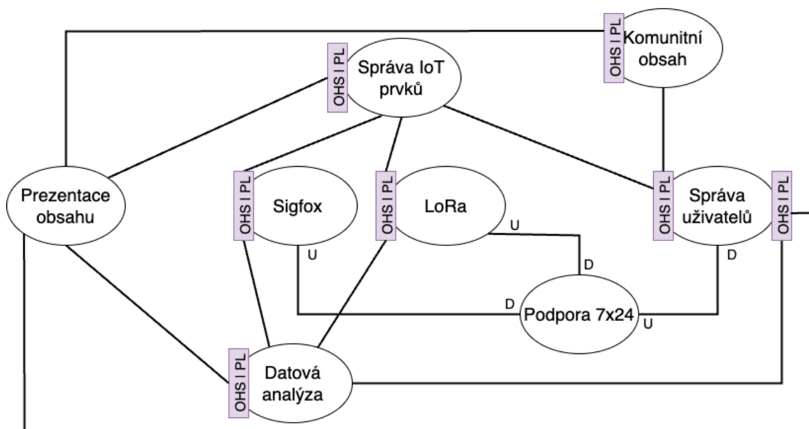
Obrázek 4.3 - Kontextová mapa
