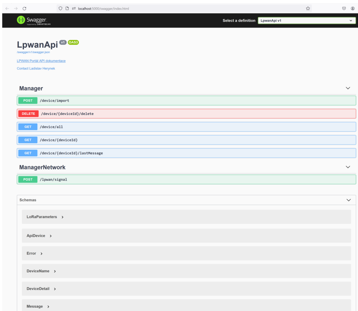
Obrázek 4.12 - OpenAPI specifikace
