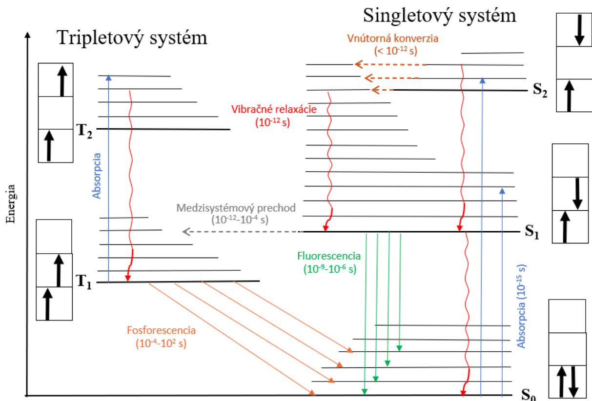
Obr. 3: Jabloňského diagram
