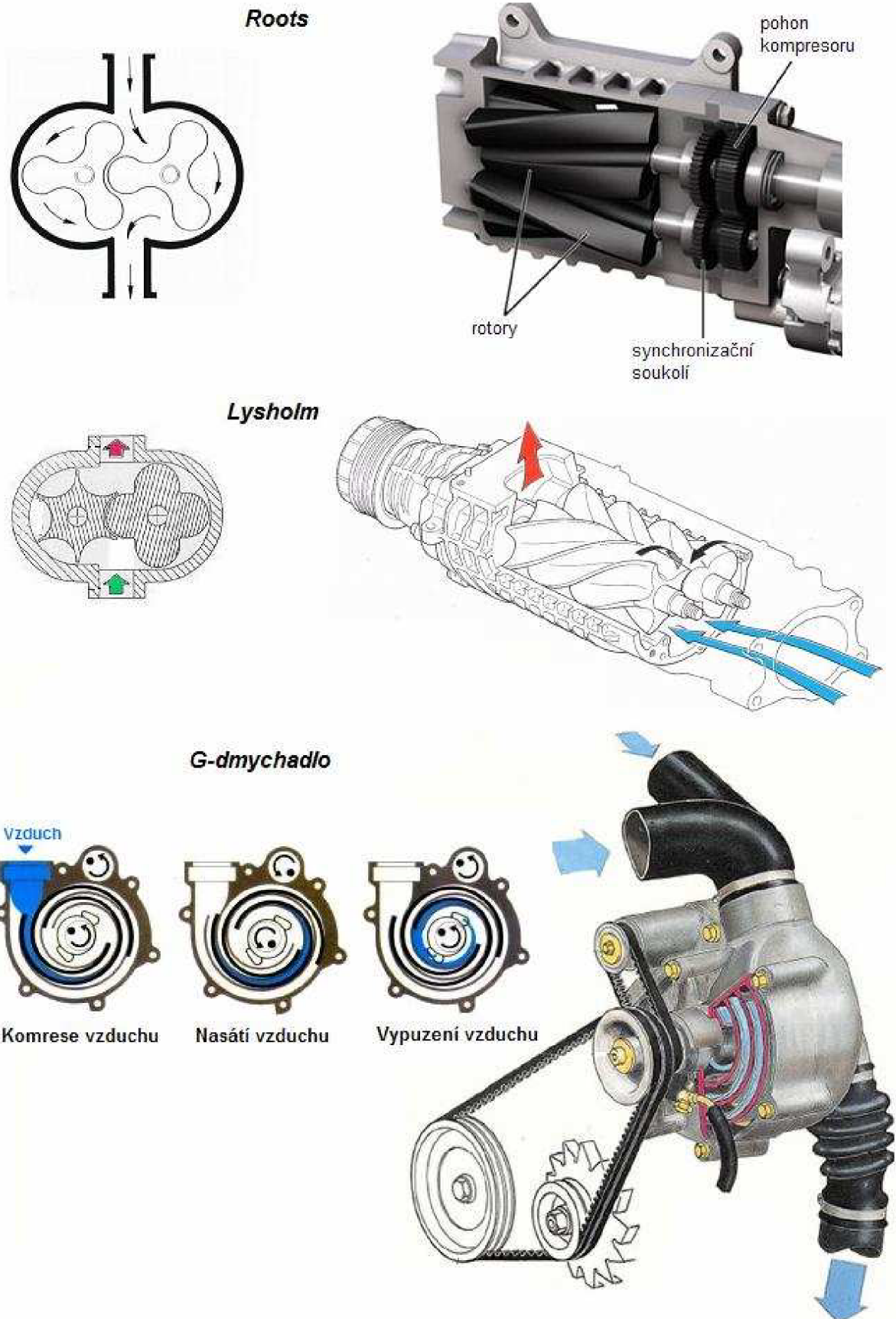
Obr. 5.3 Objemová dmychadla
