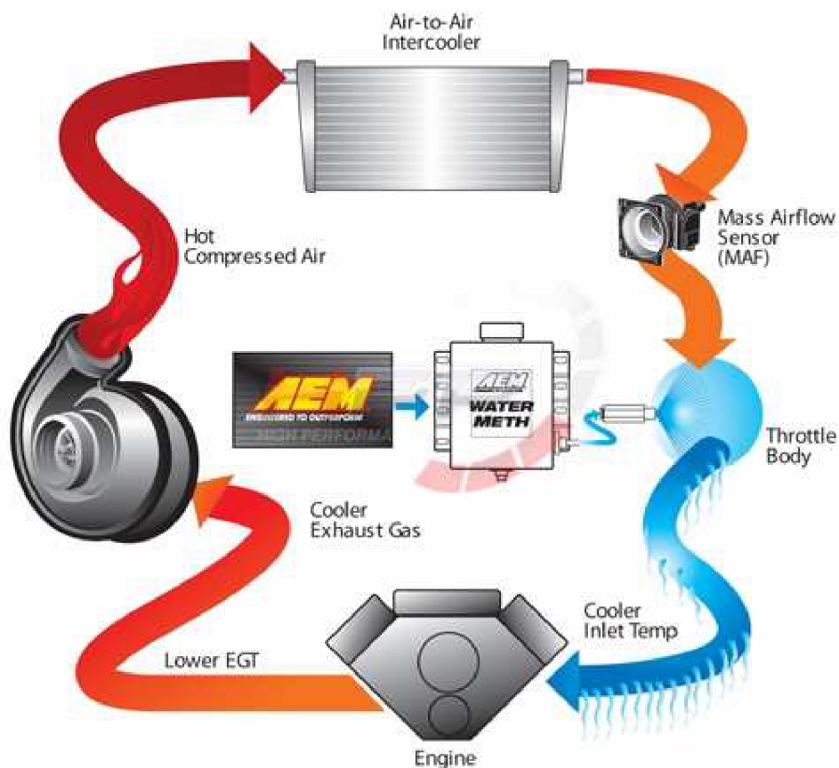
Obr. 6.2 Uspořádání systému vstřikování vody [41]
