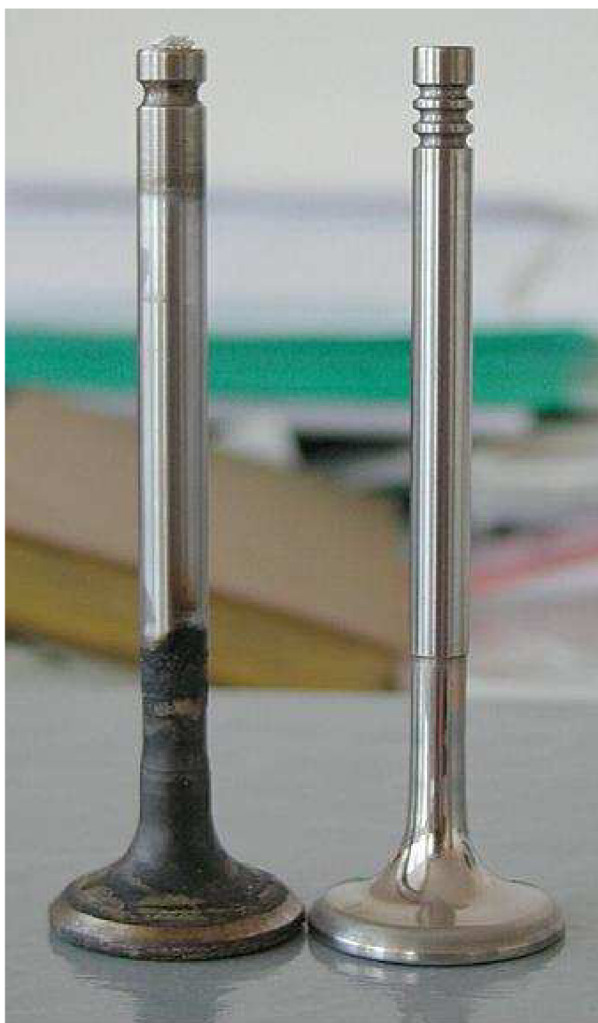
Obr. 4.8 Výfukový ventil Škoda Favorit a vedle upravený ze Škody Felicia [14]
