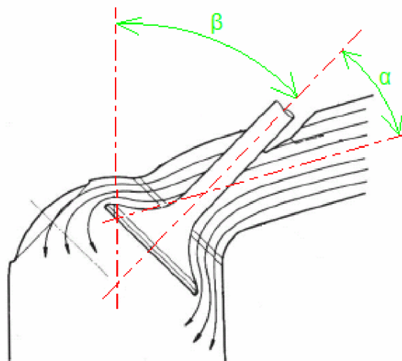
Obr. 4.2 Poloha ventilu a kanálu vůči ose válce
