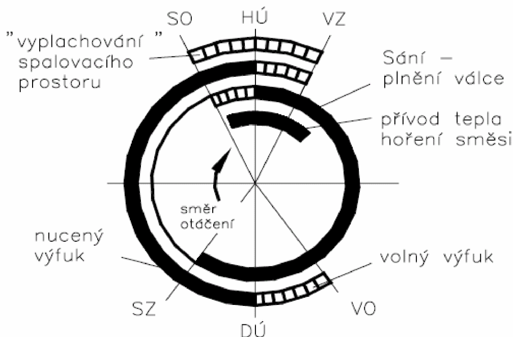
Obr. 4.5 Úhlový diagram rozvodu [16]
