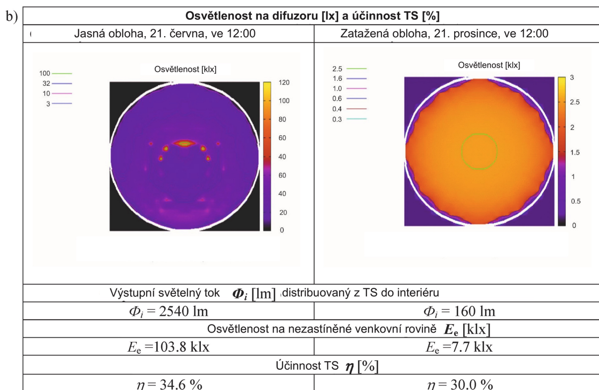
Obr. 4.11 HOLIGILM simulace osvětlenosti pro světlovod o průměru D = 0.3 m, délka L = 3 m a odraznost tubusu \rho = 0.90 ; simulováno pro jasnou oblohu (21. června, 12:00) a zataženou oblohu (21. prosince, 12:00) a) Osvětlenost [lx] na referenční rovině 2 m pod světlovodem b) Osvětlenost [lx] na difuzoru světlovodu určené pro výstupní světelný tok \Phi_i [lm], venkovní horizontální osvětlenost E_e [klx] a účinnost světlovodu \eta [%].
