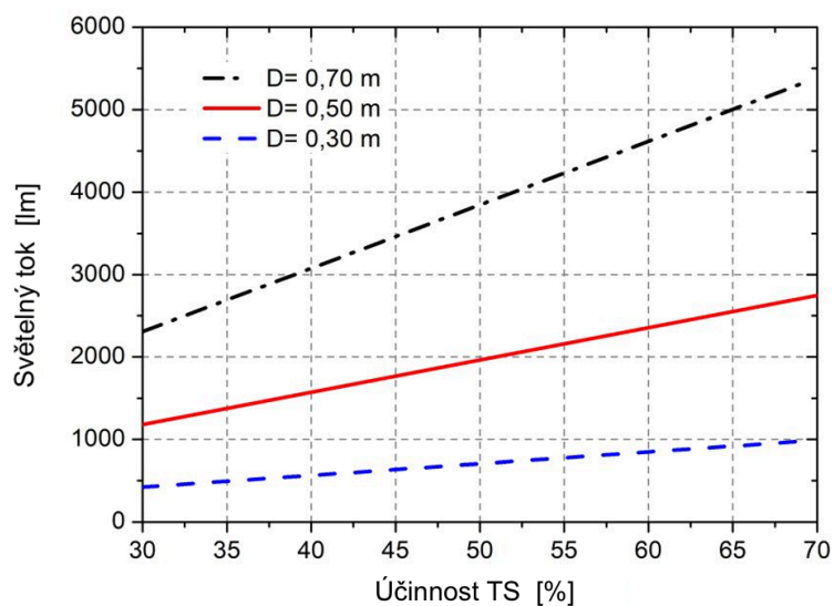
Obr. 4.14 Světelný tok \Phi_i vstupující do interiéru z tubusového světlovodu (TS), D – průměr tubusu světlovodu.
