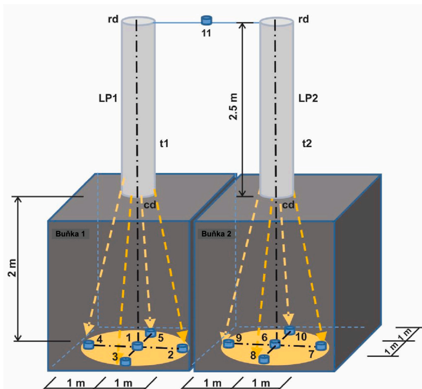
Obr. 3.2 Schéma instalace luxmetrů pod světlovody
