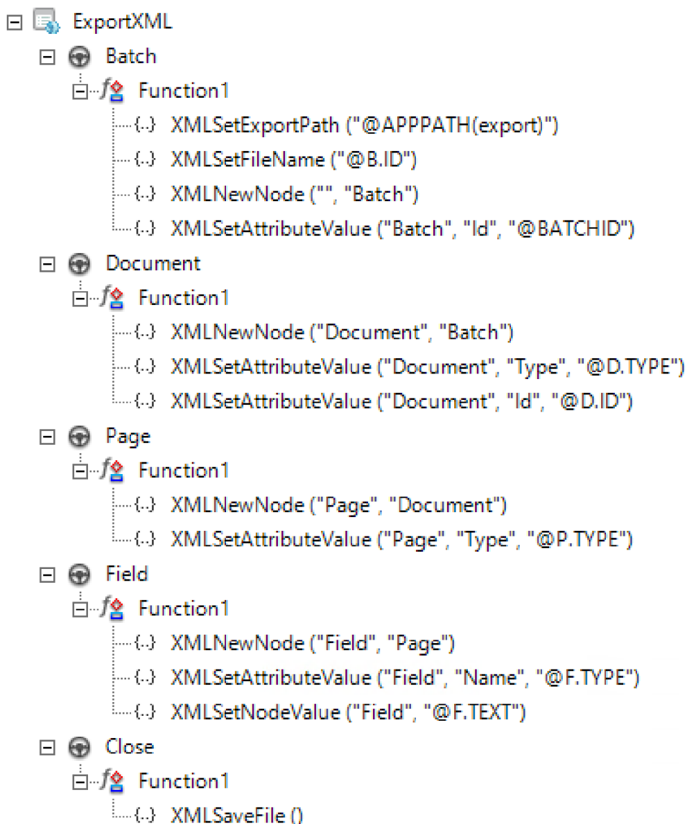
Obrázek 20 Ukázka funkce pro export dat xml formátu (vlastní zdroj)
