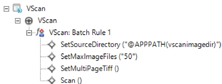
Obrázek 12 Ukázka upraveného setu pravidel pro import dokumentů (vlastní zdroj)
