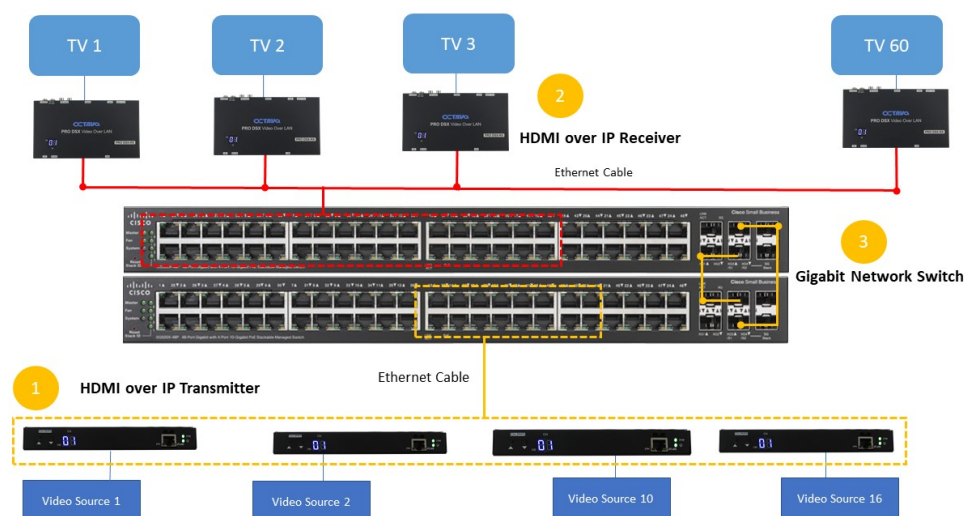
Obr. 2.1: Obrázok znázorňuje zapojenie prijímačov a vysielačov do ethernetovej siete [14]. Žltou farbou je znázornené zapojenie vysielačov do ethernetového prepínača, typicky pomocou Cat 5e/6 kabeláže. Červenou farbou je zobrazené pripojenie prijímačov do ethernetového prijímača, aby mohli prijímať pakety obsahujúce snímky zo vstupného videa vysielačmi. Číslami pri názvoch video zdrojov (Video Source X) je vyjadrená škálovateľnosť v smere pridávania nových video zdrojov. Rovnako tak pri číslach prijímačov (TV X) je vyjadrená škálovateľnosť v smere pridávania nových koncových staníc.
