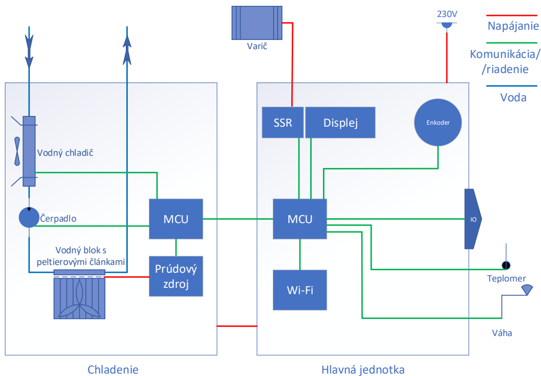
Obr. 3.2: Blokovaná schéma zapojenia
