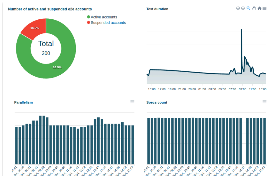
Obr. 12: Komponenta Dashboard
