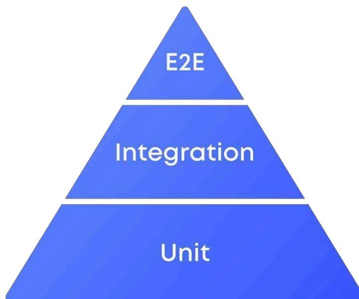
Obr. 5: Testovací pyramida [21]
