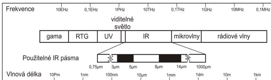
Obr. 3.1 Elektromagnetické spektrum
