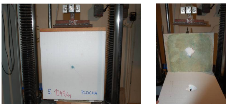
Obr. 10 Vzorek připravený ve zkušebním lisu a po ukončené zkoušce
